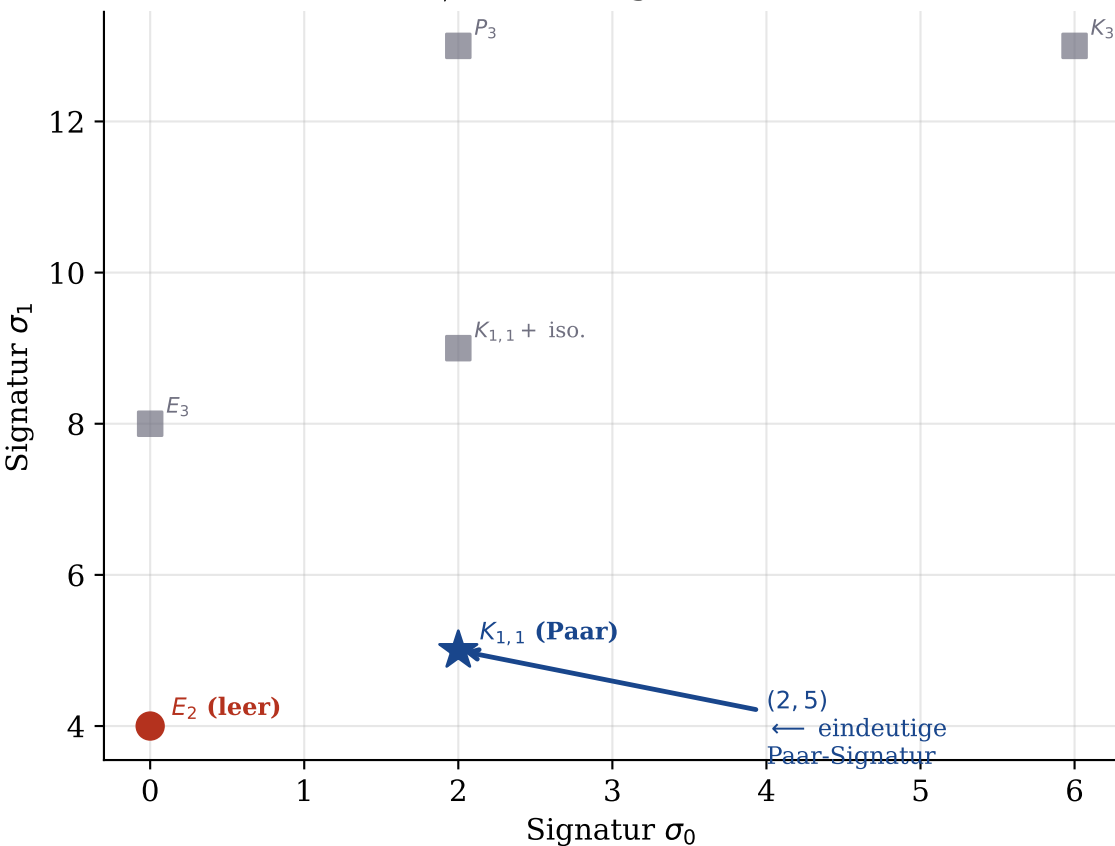
(b) Signaturraum ( \sigma_0, \sigma_1 ) K_{1,1} eindeutig bei (2, 5)
