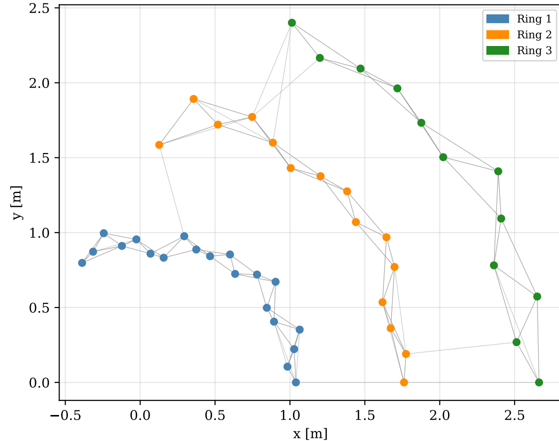
(b) k-NN Graph (k=4) der Punktwolke
