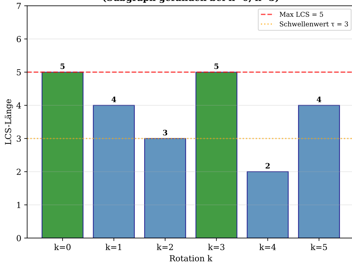
(b) LCS-Wert je Rotation (Subgraph gefunden bei k=0, k=3)
