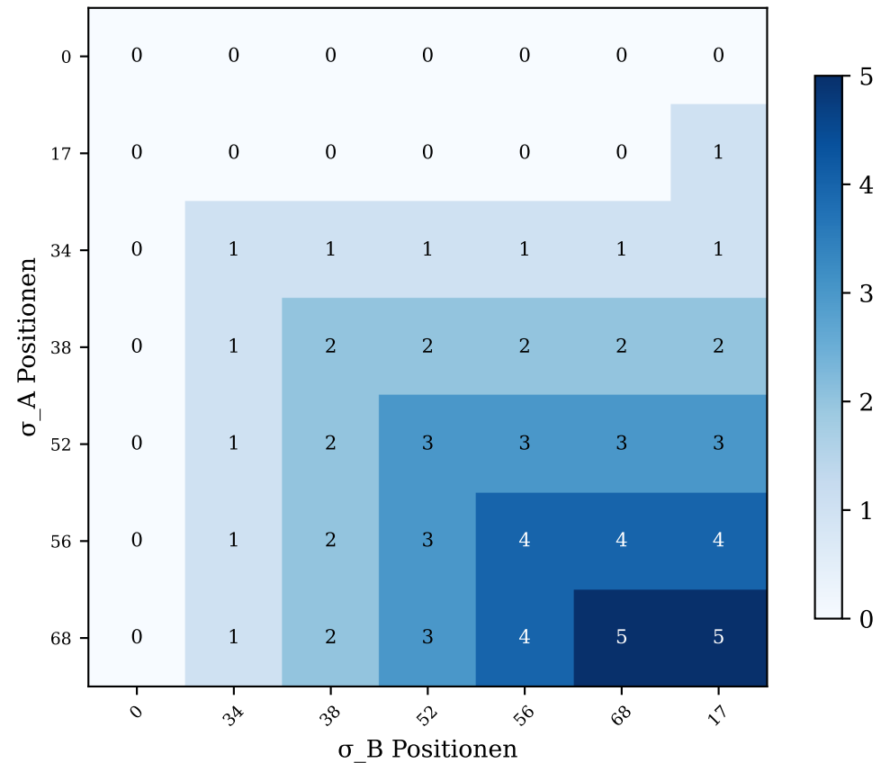
(a) LCS-DP-Tabelle |LCS| = 5 → Subgraph erkannt!
