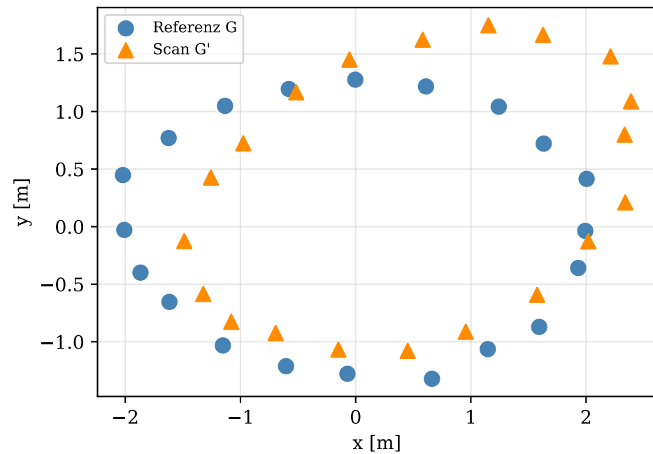
(a) Vor Registrierung (25° Rotation, 0.58 m Translation)
