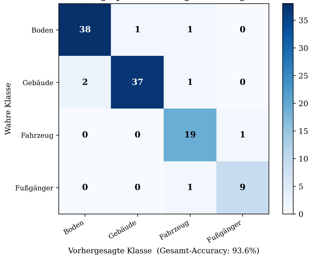
(b) Konfusionsmatrix (Subgraph-basierte Segmentierung)
