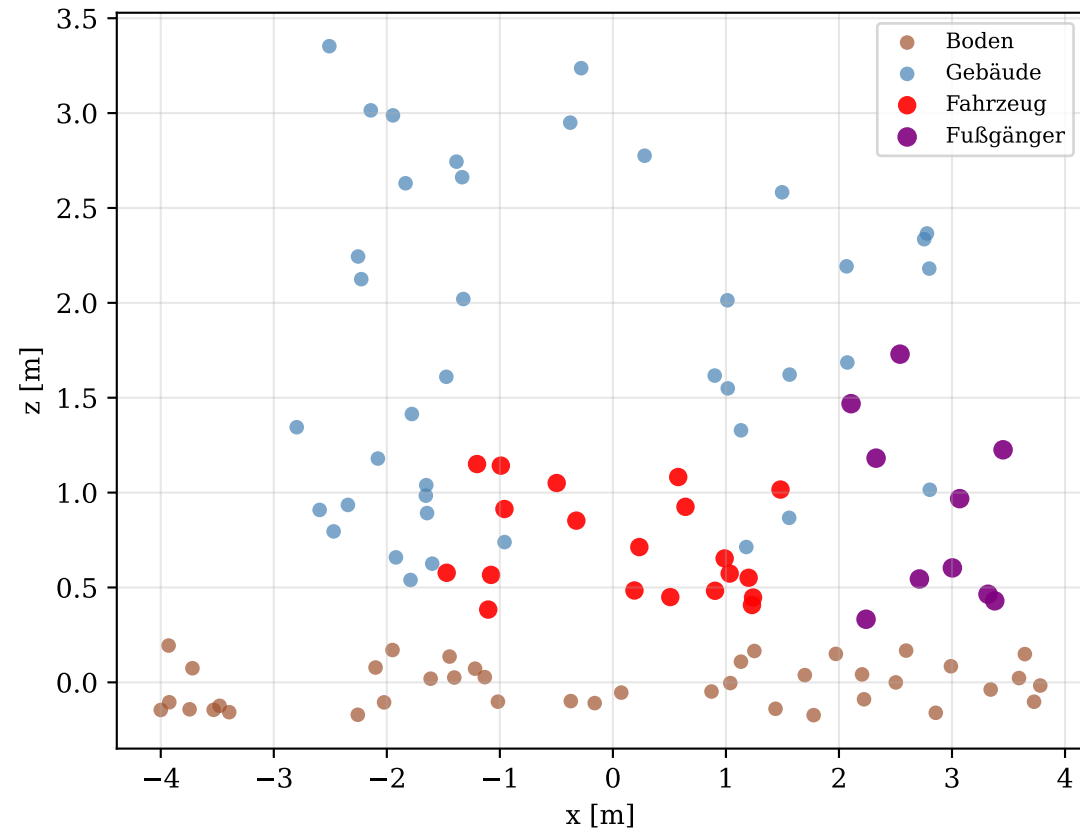
(a) Subgraph-Segmentierung der LiDAR-Punktwolke
