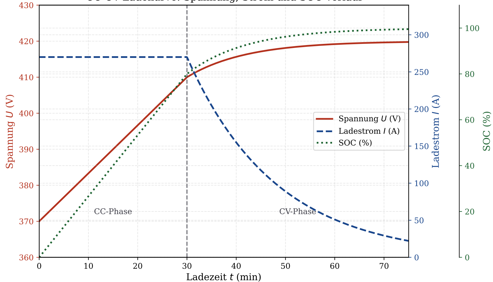
CC-CV-Ladekurve: Spannung, Strom und SOC-Verlauf
