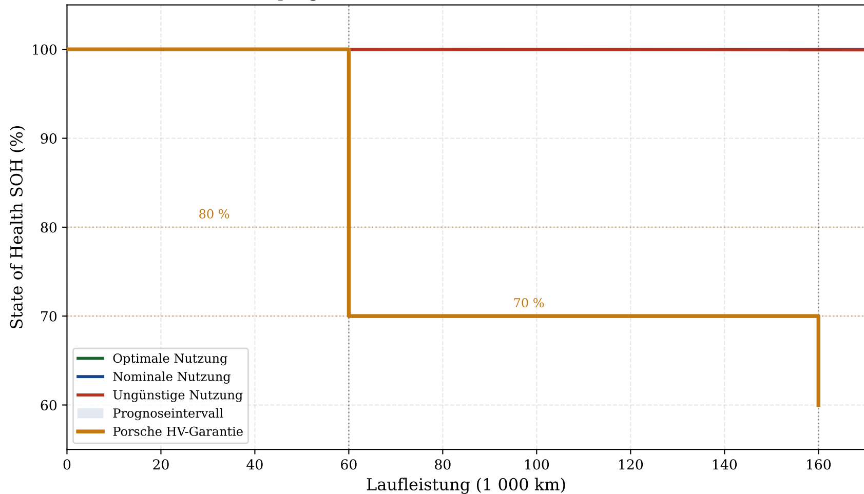
Modellprognose vs. Porsche HV-Batterie-Garantiekurve
