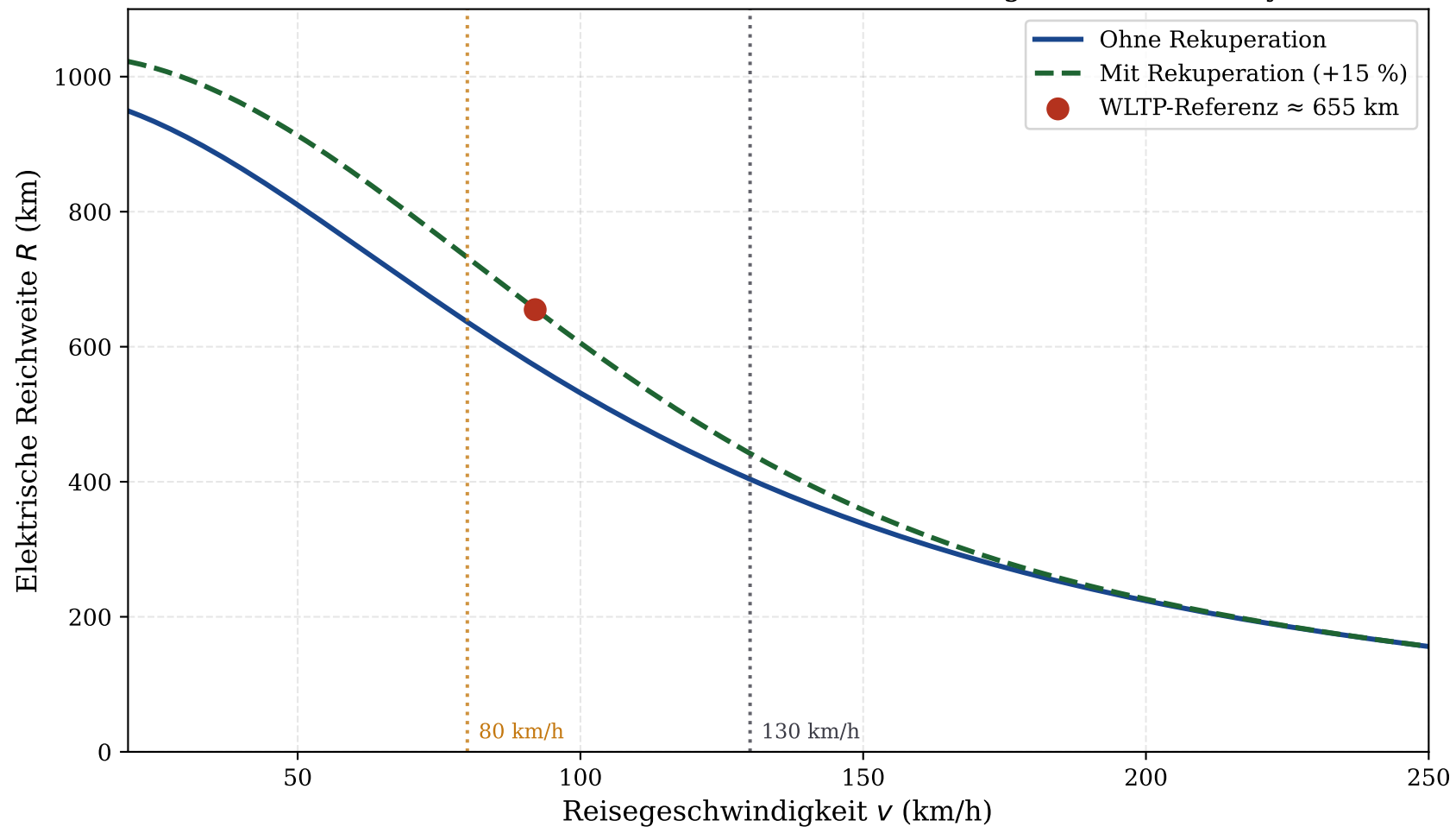
Elektrische Reichweite als Funktion der Geschwindigkeit (Porsche Taycan)
