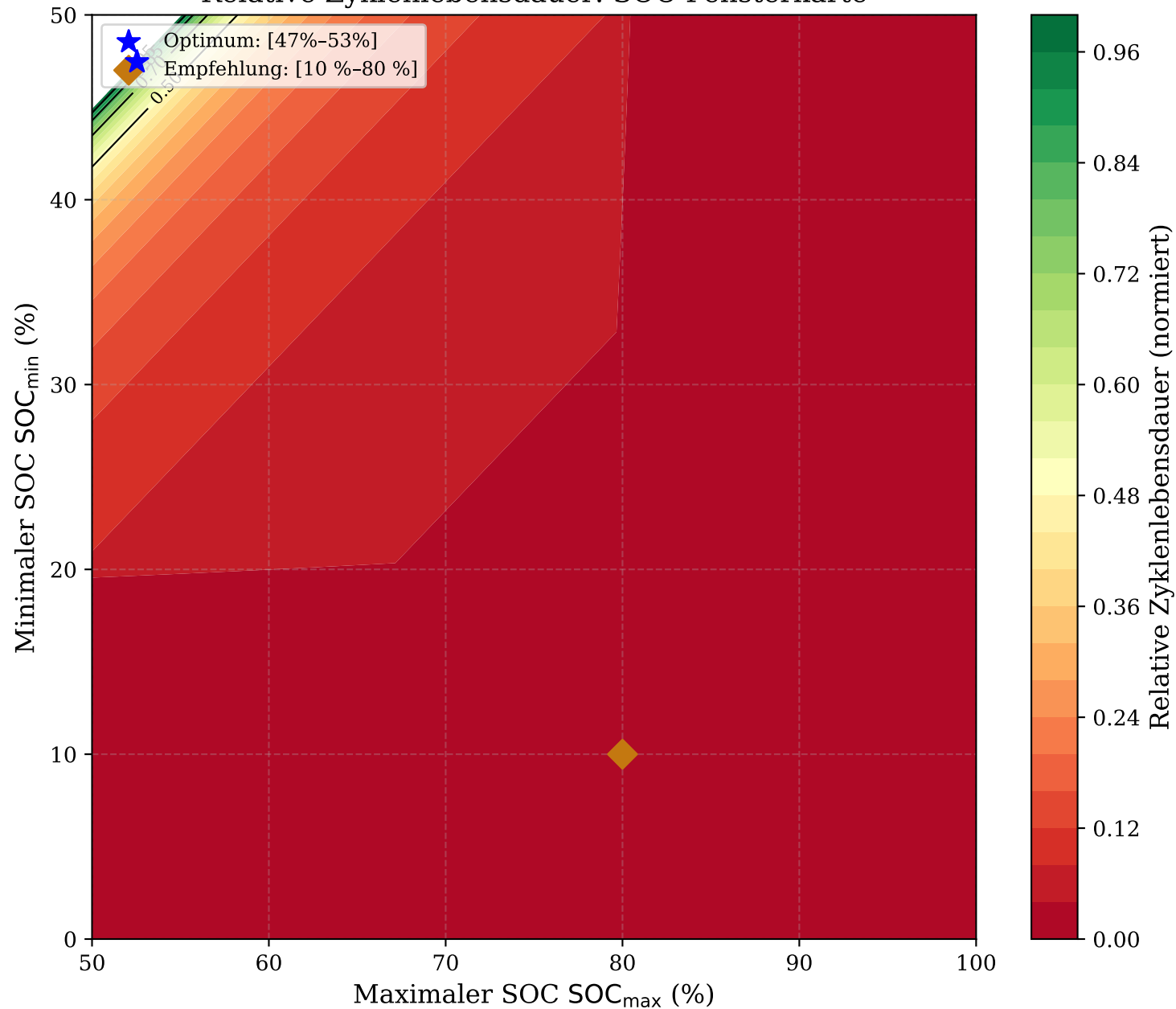
Relative Zykluslebensdauer: SOC-Fensterkarte
