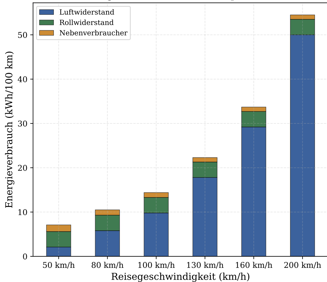
Energieverbrauch nach Komponenten
