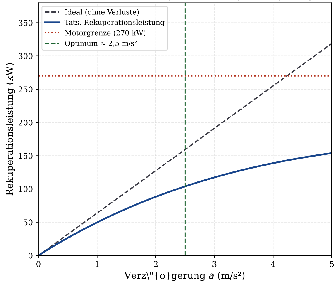
Rekuperationsleistung vs. Fahrzeugverzögerung
