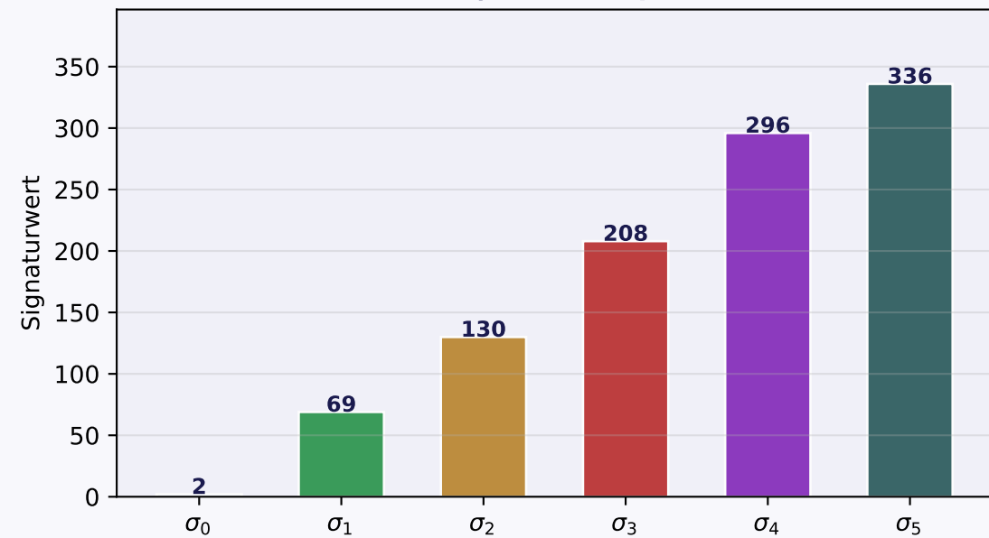
Subgraph-Algorithmus auf Fehlersyndrom-Graphen Signaturen \sigma_j = \sum_i A_{ij} \cdot 2^i + j \cdot 2^n des Syndrom-Graphen
