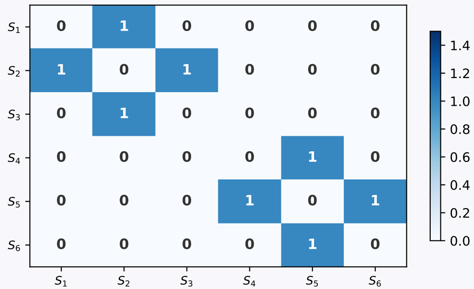
Syndrom-Adjazenzmatrix A_S (Fehlerketten als Kanten)
