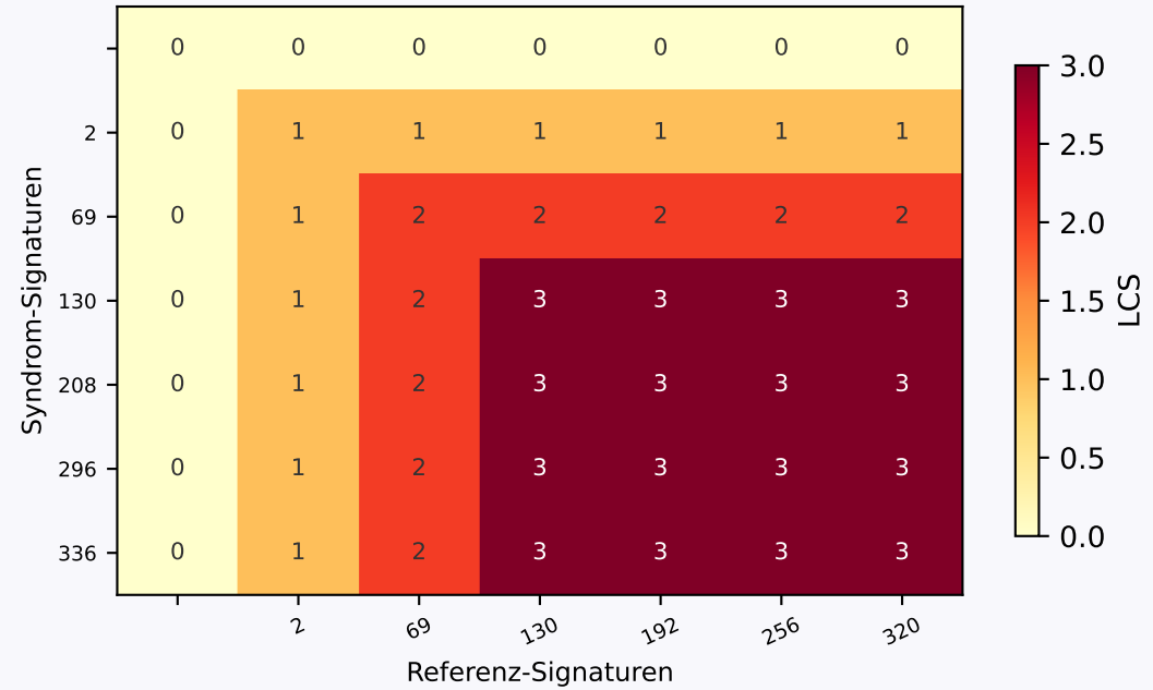
LCS-DP-Matching: |\text{LCS}| = 3 Fehlermuster erkannt? Ja ( \geq 2 )
