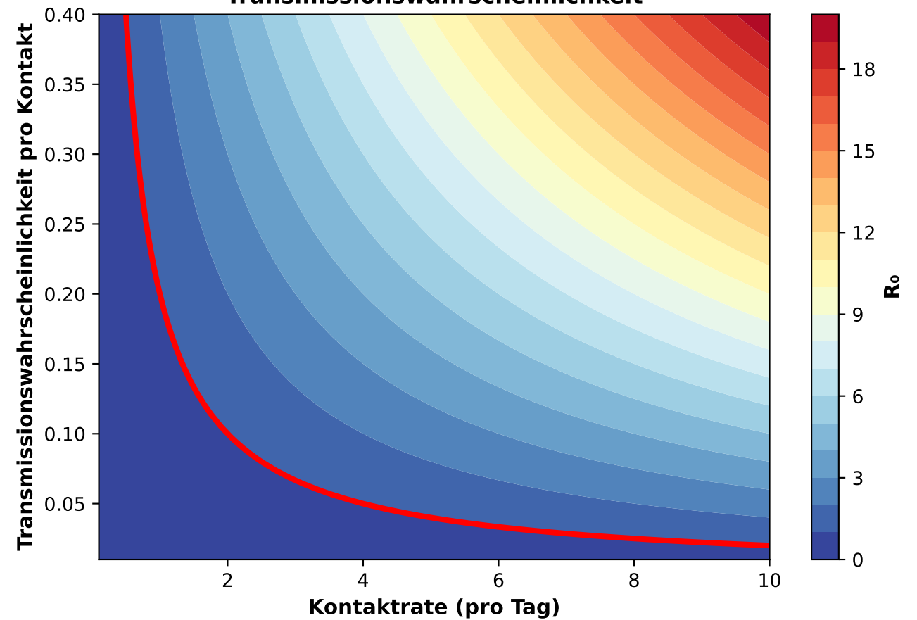
R_0 als Funktion von Kontaktrate und Transmissionswahrscheinlichkeit
