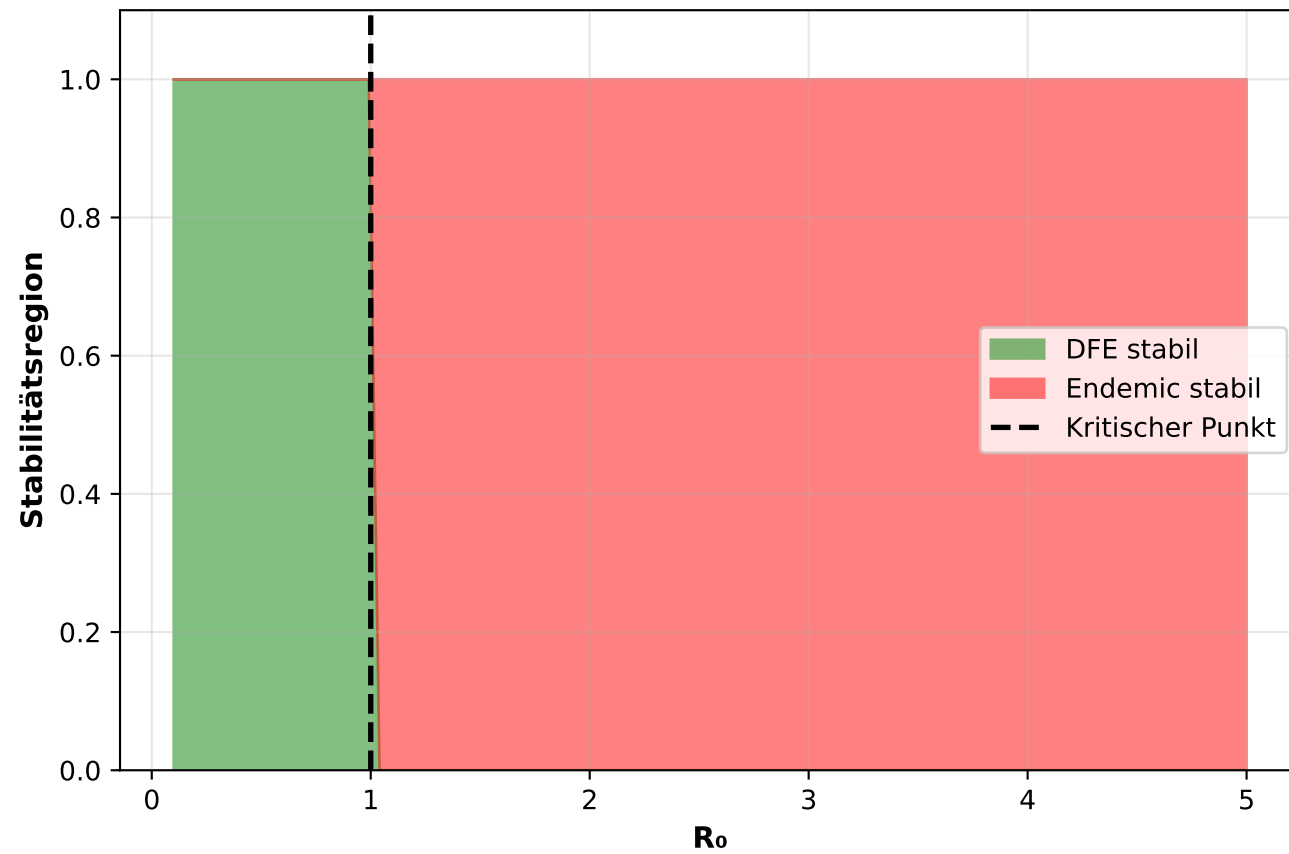
Stabilitätskarte: DFE vs. Endemie
