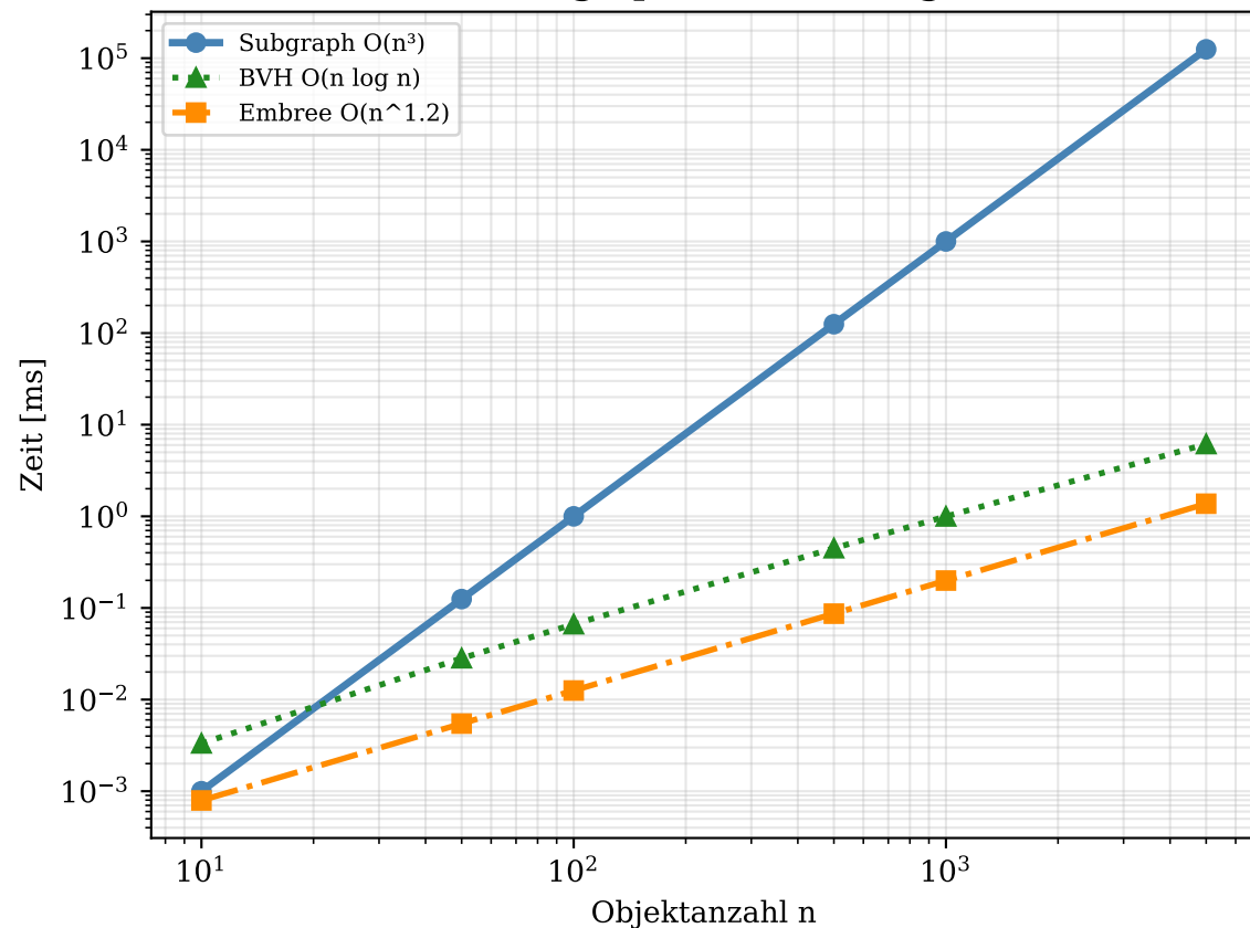
(b) Praktische Laufzeit [ms] (Szenegraph-Traversierung)
