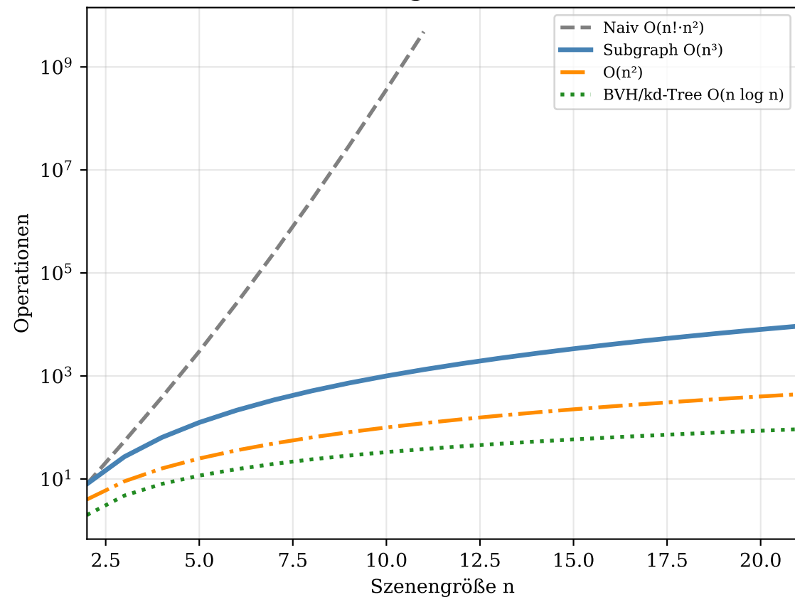
(a) Zeitkomplexität im Vergleich (log-Skala)
