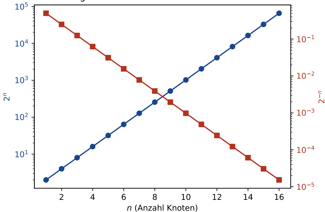
Divergenz von 2^n und 2^{-n} mit wachsendem n
