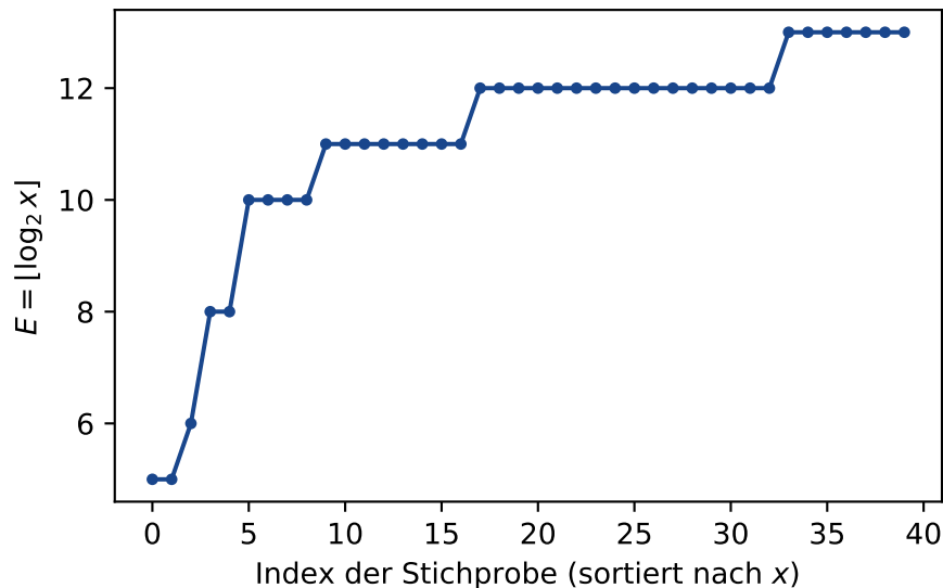
Exponentenanteil (Skaleninformation)
