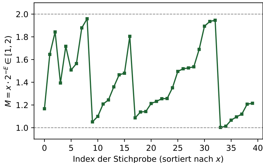
Mantissenanteil (Forminformation)
