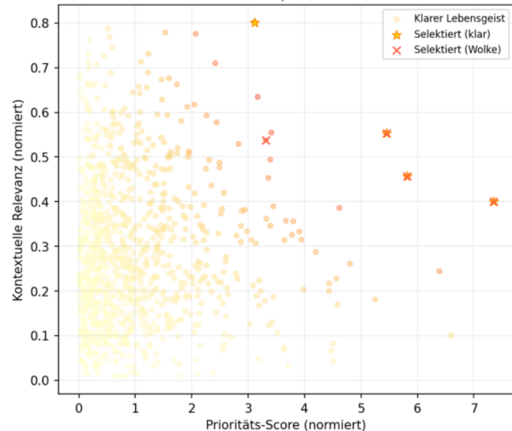
Thalamus-ARAS: Selektiver Informations-Gateway
