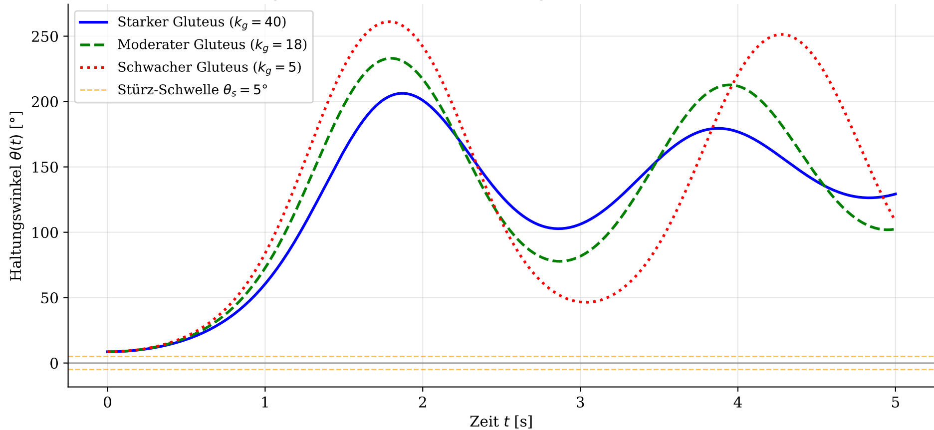
Abbildung 7: Posturale Stabilisierung - Invertiertes Pendelmodell
