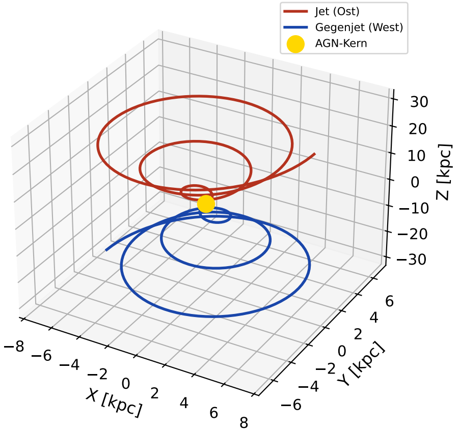
3D-Jet-Trajektorie (helikale Präzession)
