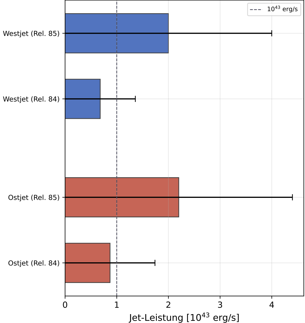
Kinetische Jet-Leistungen (nach Skalenrelationen)
