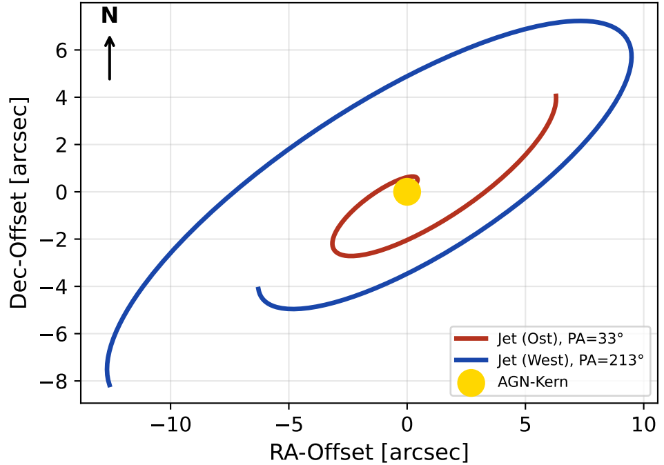
Himmelsprojektion \psi = 33^\circ, \phi = 14^\circ, i = 71^\circ
