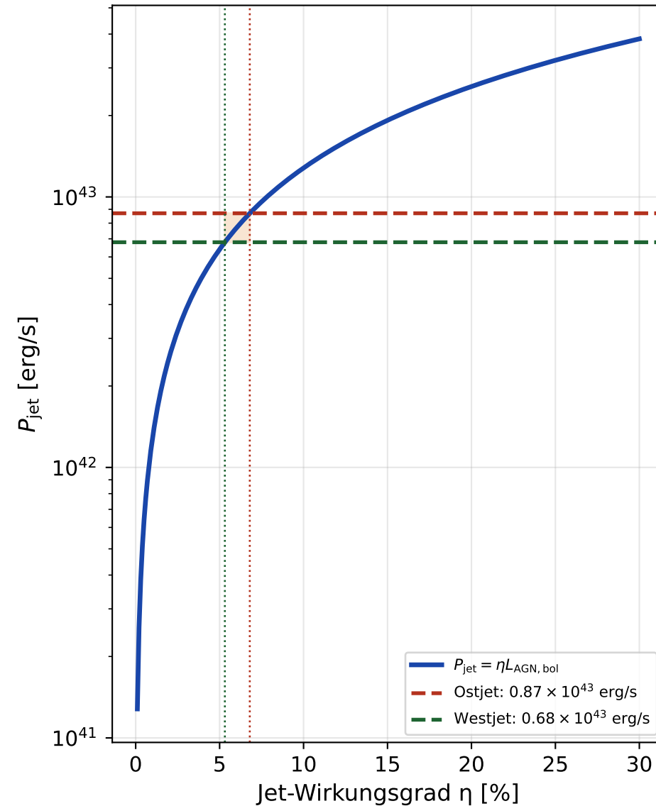
Jet-Wirkungsgrad (Kopplung an AGN-Leuchtkraft)
