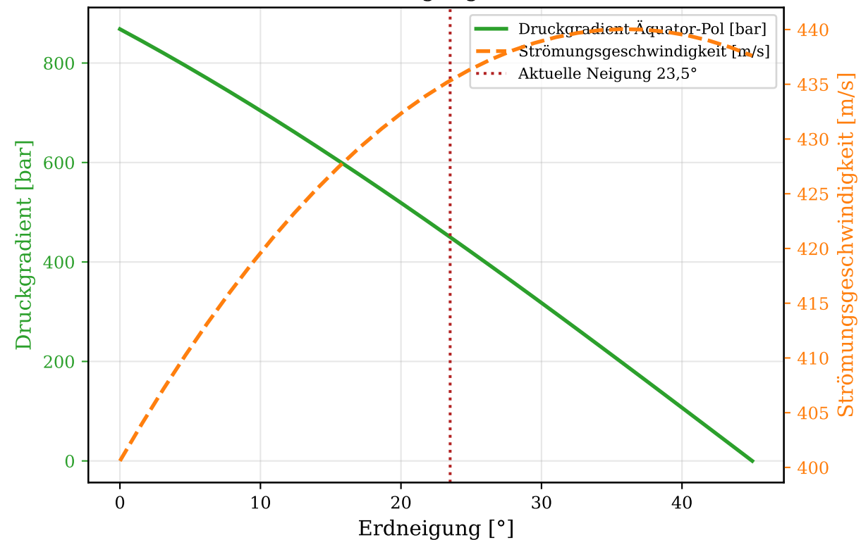
Druckgradient und Strömungsgeschwindigkeit vs. Erdneigungswinkel
