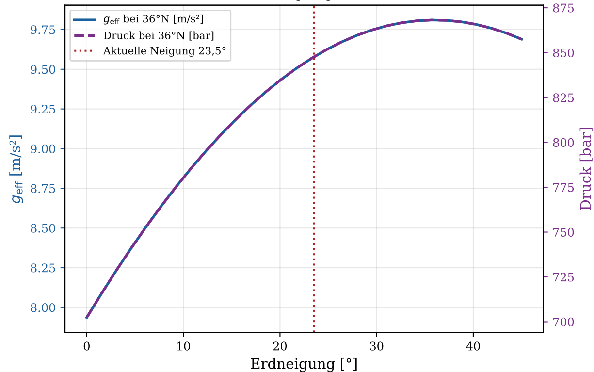
Effektive Gravitation und Druck bei 36°N vs. Erdneigungswinkel
