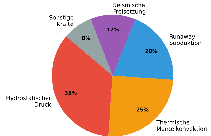
Antriebskräfte der Sintflut-Tektonik (Energieanteile, schematisch)
