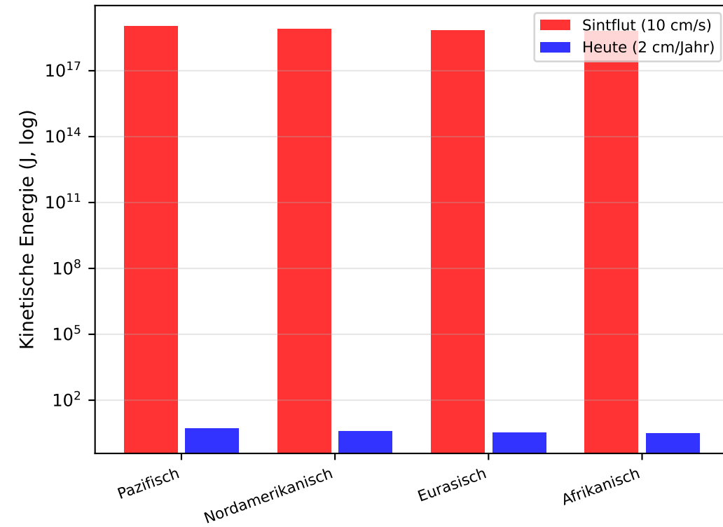
Antriebskräfte der Sintflut-Tektonik (Energieanteile, schematisch)
