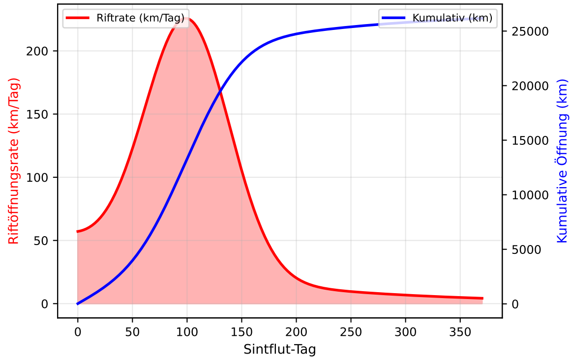
Kontinentalrift-Öffnungsrate am Atlantik
