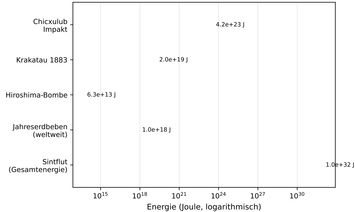
Vergleich Energiequellen (Sintflut dominiert)
