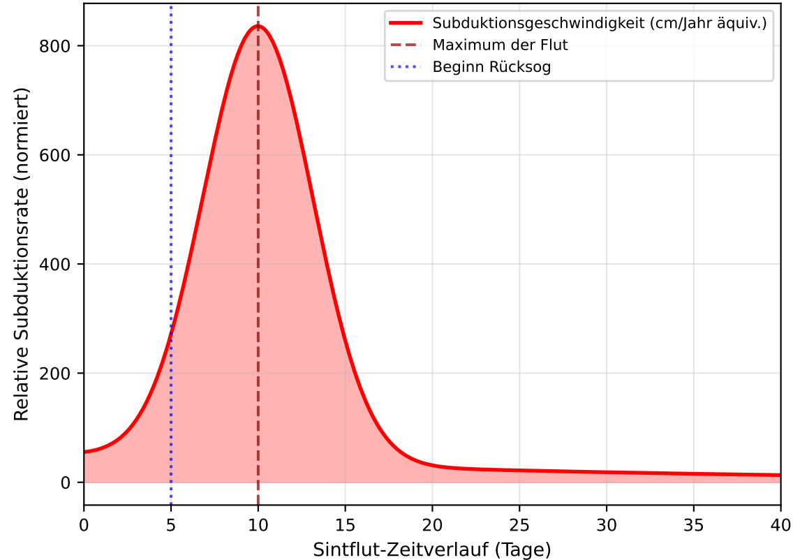
Zeitverlauf der Subduktionsgeschwindigkeit
