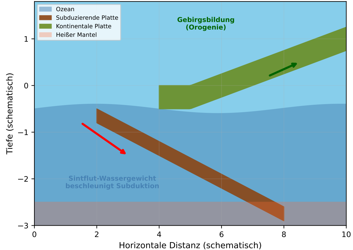
Schematischer Querschnitt: Sintflut-Subduktionszone
