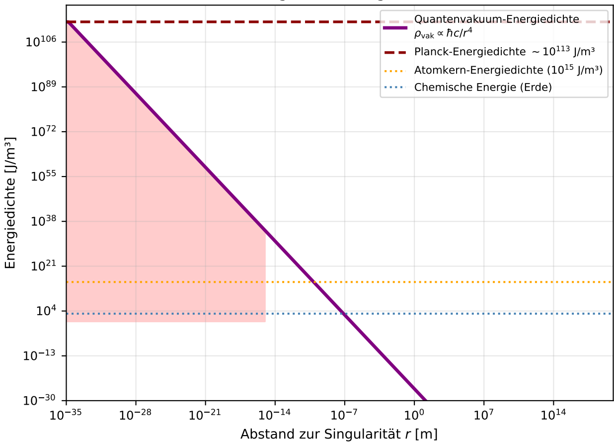
Quantenvakuum-Energiedichte: Divergenz zur Singularität
