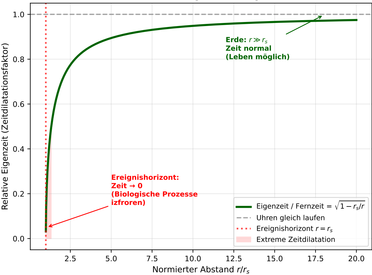
Gravitationszeitdilatation: Zeit kommt zum Erliegen am Ereignishorizont
