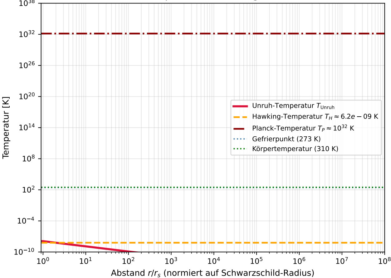
Unruh-Temperatur nahe Ereignishorizont
