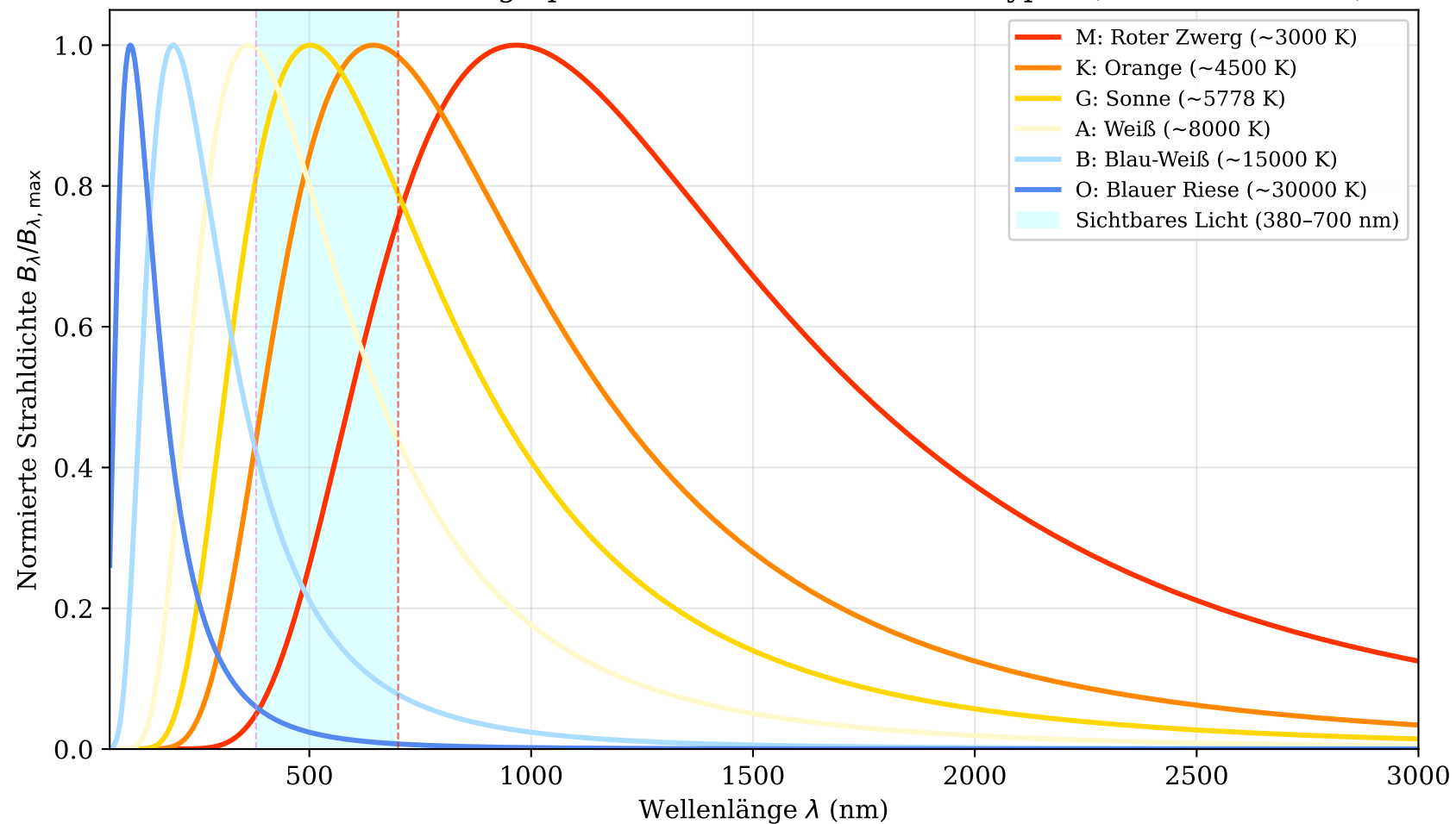
Planck'sches Strahlungsspektrum verschiedener Sterntypen (Harvard-Klassen)
