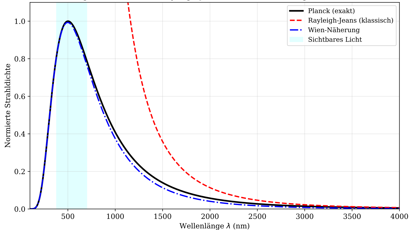
Vergleich: Planck vs. Rayleigh-Jeans vs. Wien-Näherung ( T = 5778 \text{ K} )
