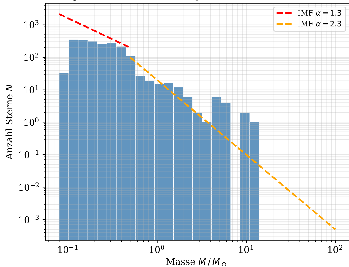
Anfangsmassenfunktion (Kroupa IMF) im simulierten Cluster
