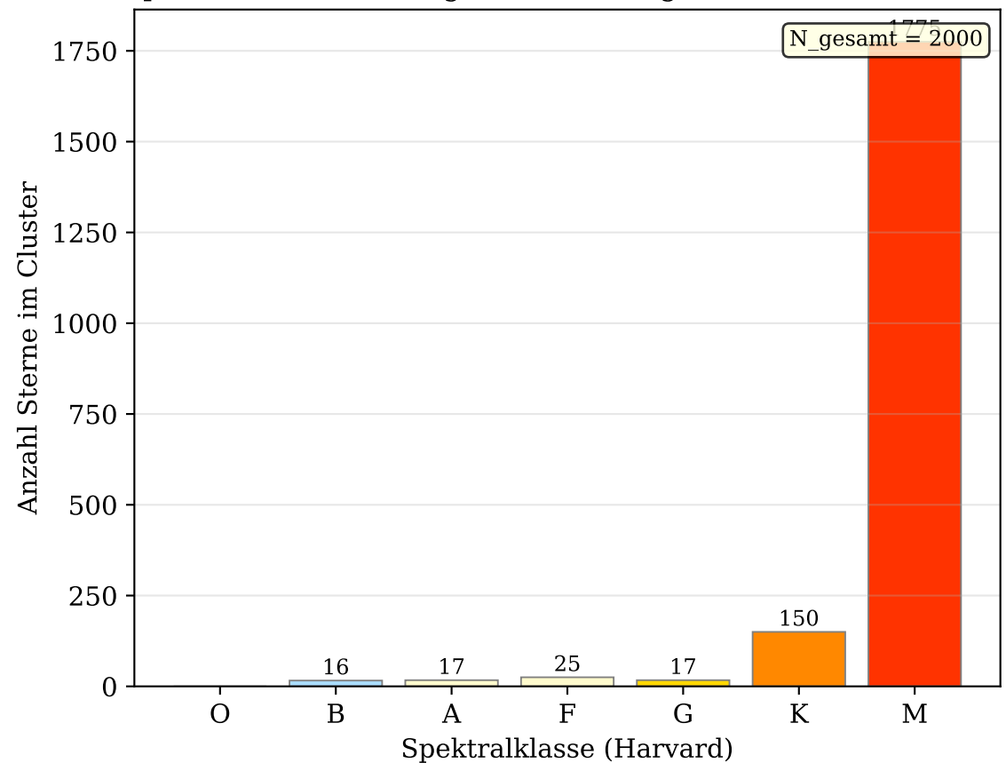
Spektralklassen-Häufigkeitsverteilung im simulierten Cluster
