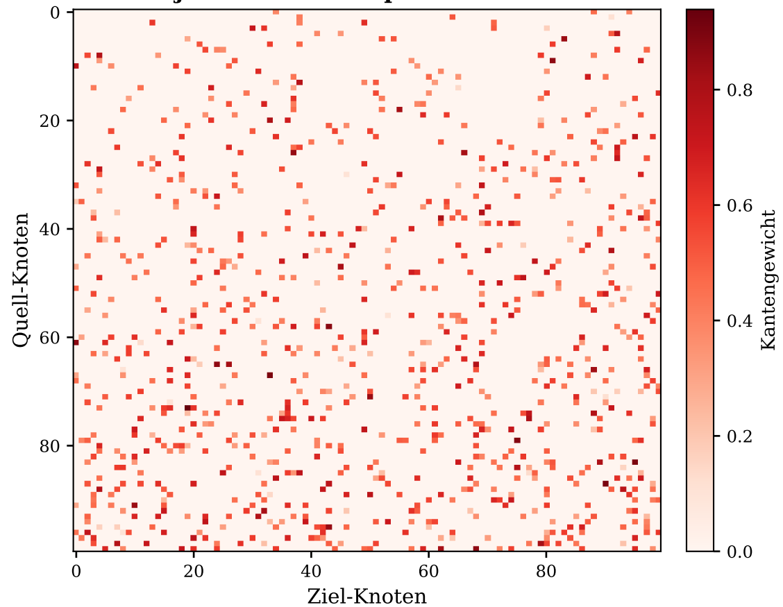
Adjazenzmatrix: Depressives Gehirn
