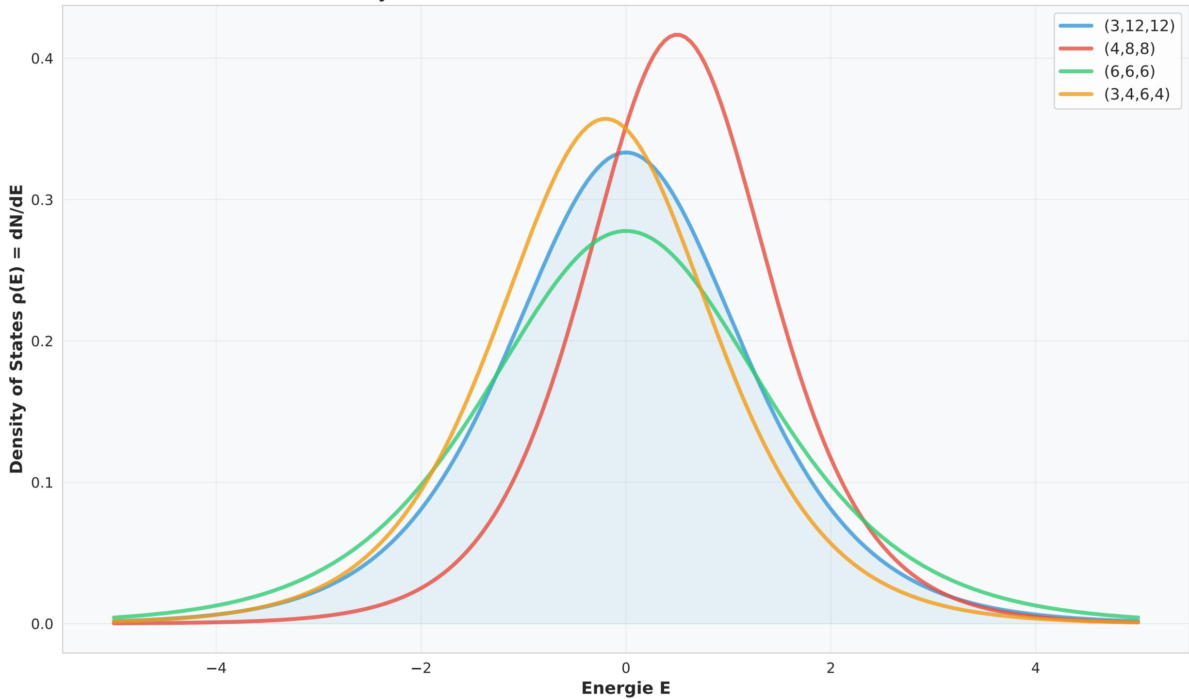
Density of States (DOS) für verschiedene Archimedean Gitter
