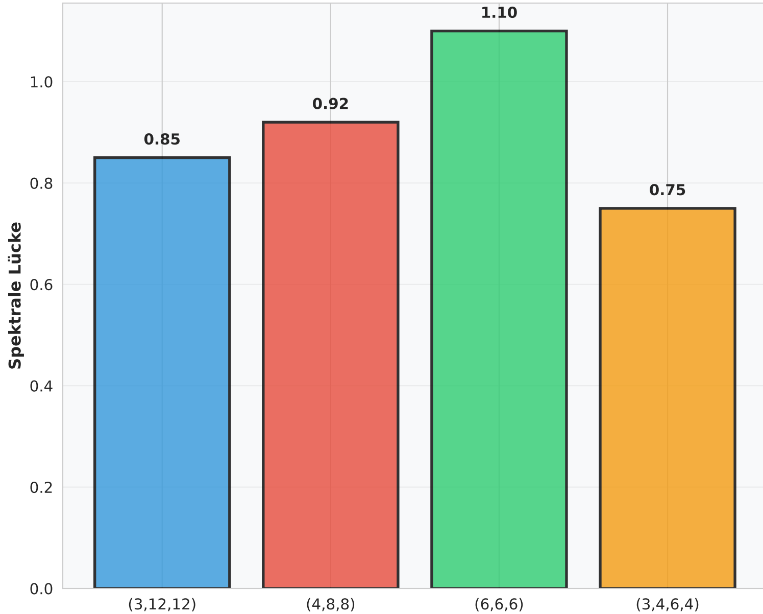
Spektrale Lücke verschiedener Archimedean Gitter
