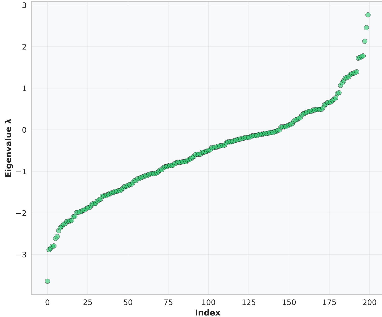
Eigenvalue Spektrum des (6,6,6) Hexagon-Gitters
