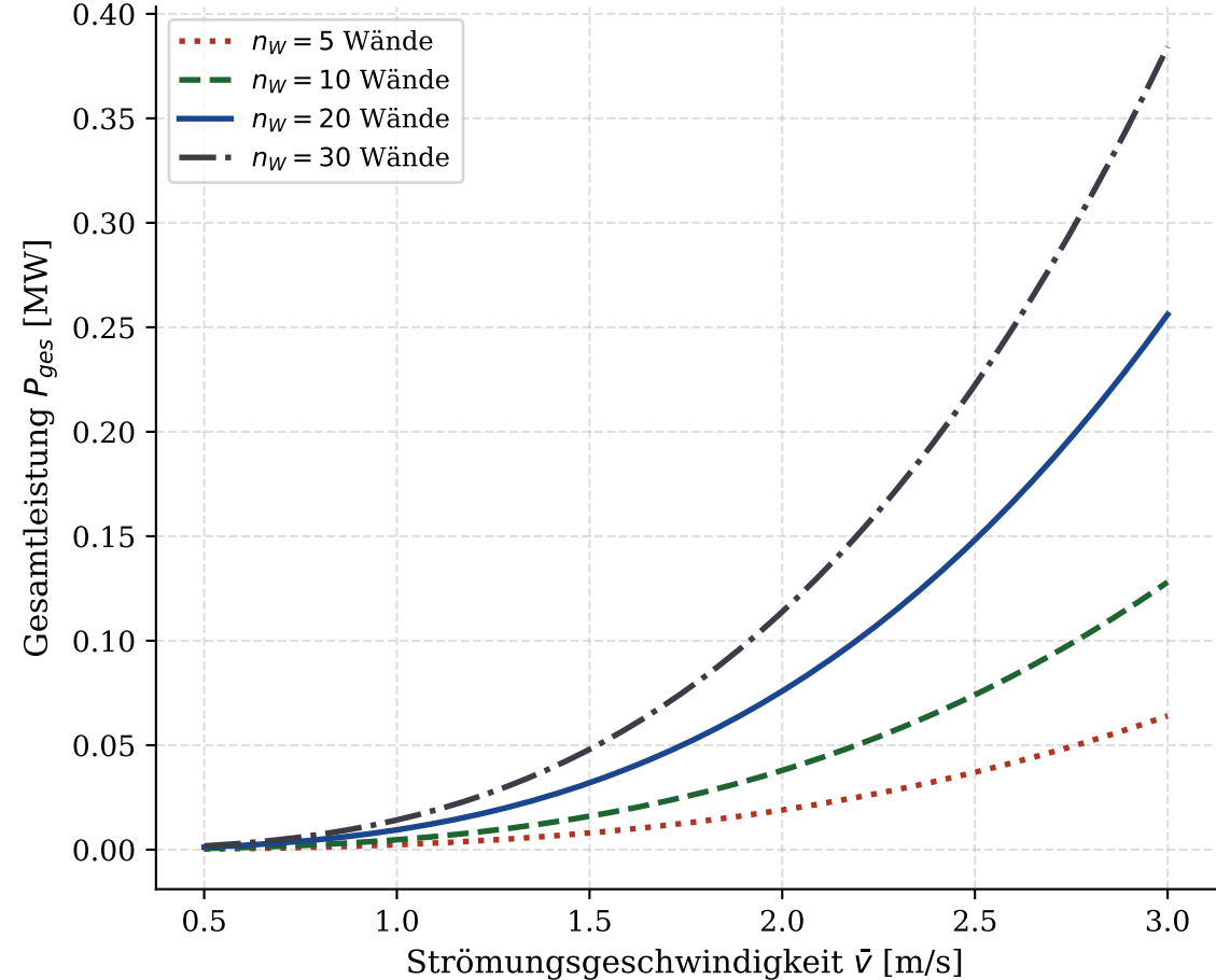
Gesamtleistung in Abhängigkeit von Strömungsgeschwindigkeit und Wandanzahl
