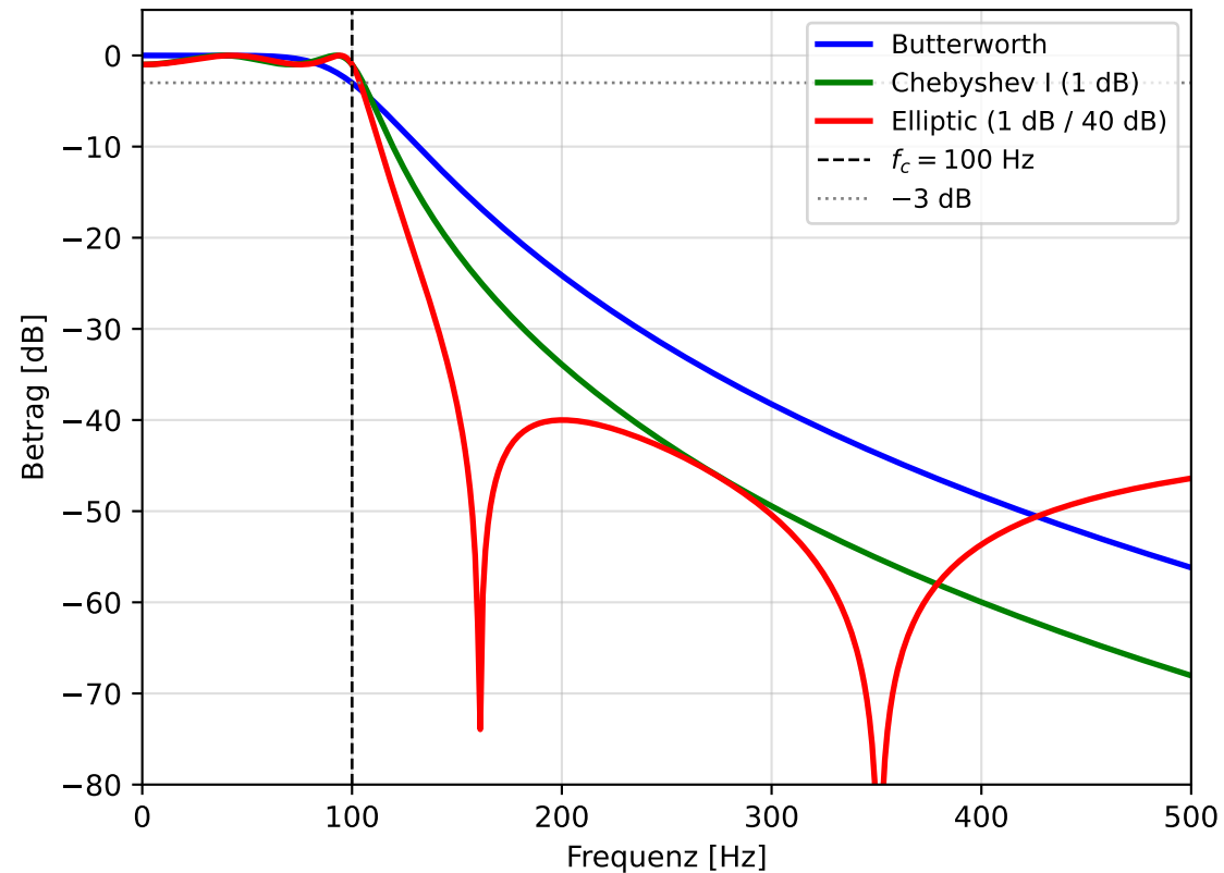
Amplitudengang
