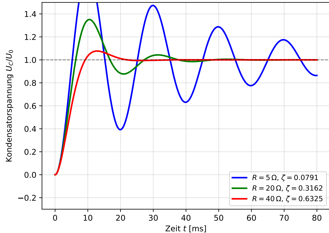
RLC-Stromkreis: Drei Dämpfungsfälle
