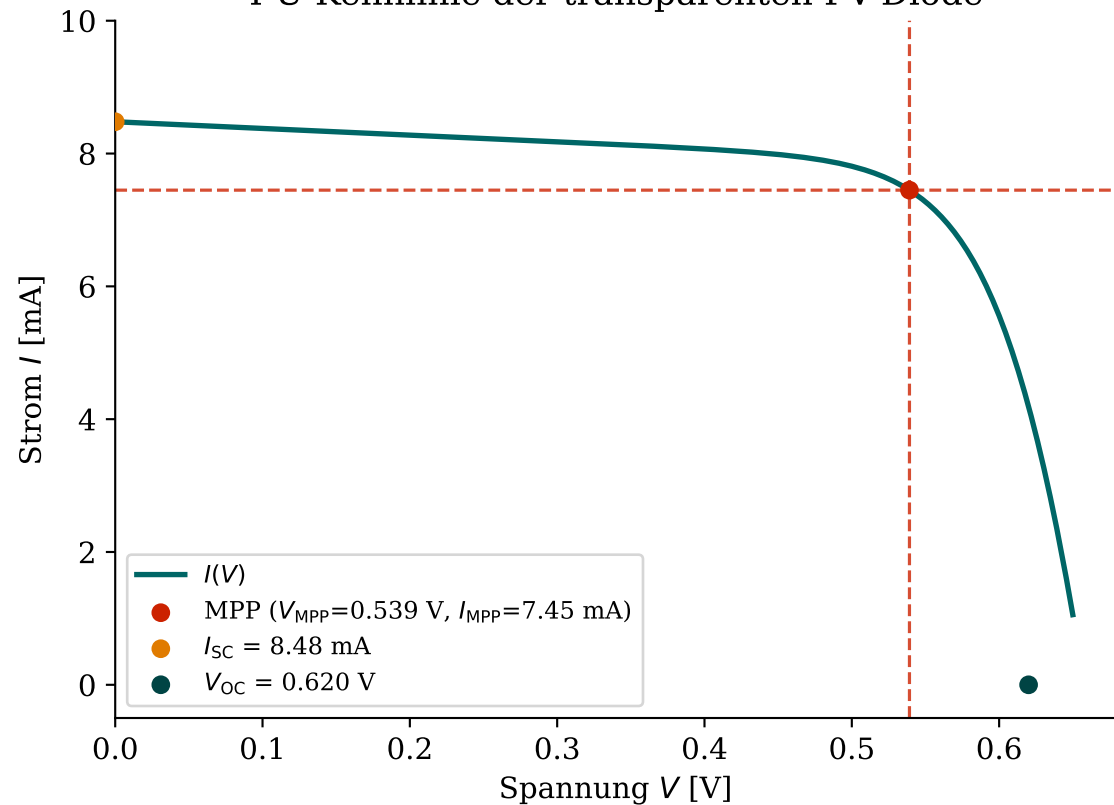
I-U-Kennlinie der transparenten PV-Diode
