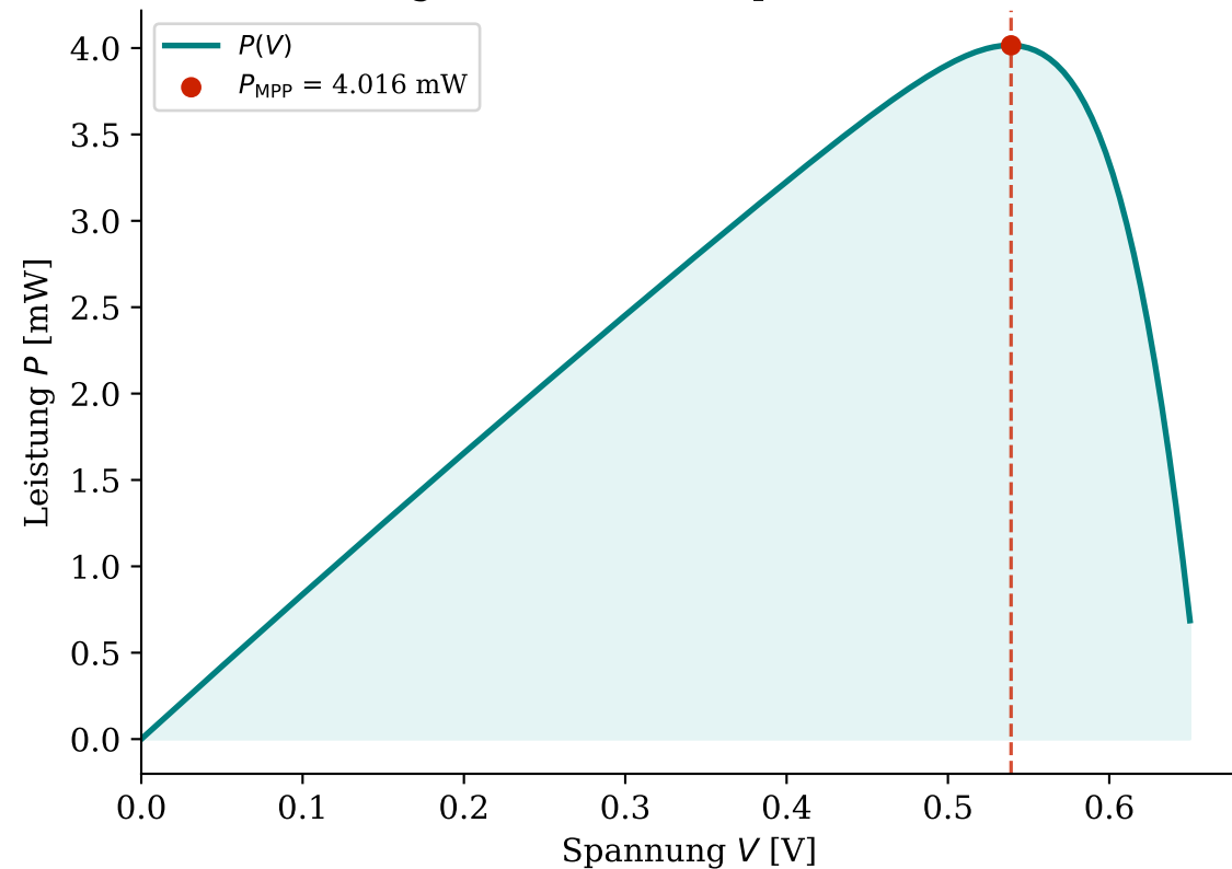
Leistungskurve der transparenten PV-Diode
