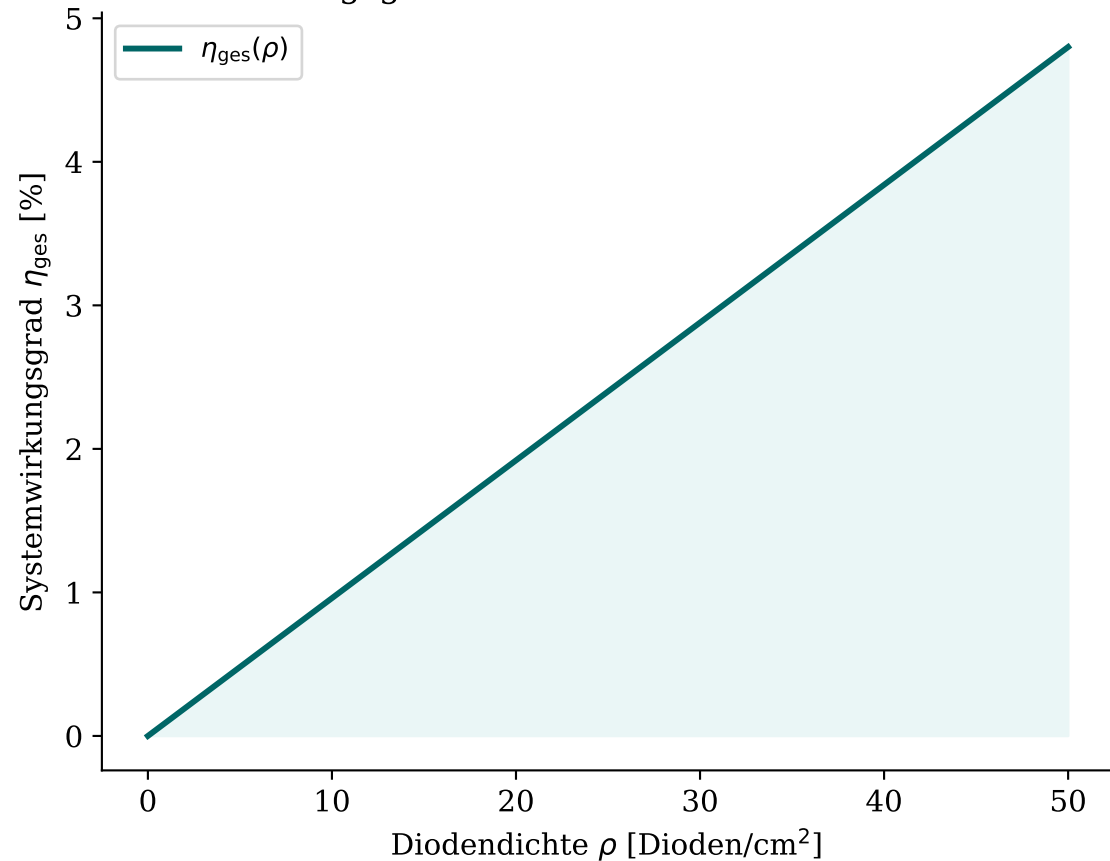
Wirkungsgrad als Funktion der Diodendichte
