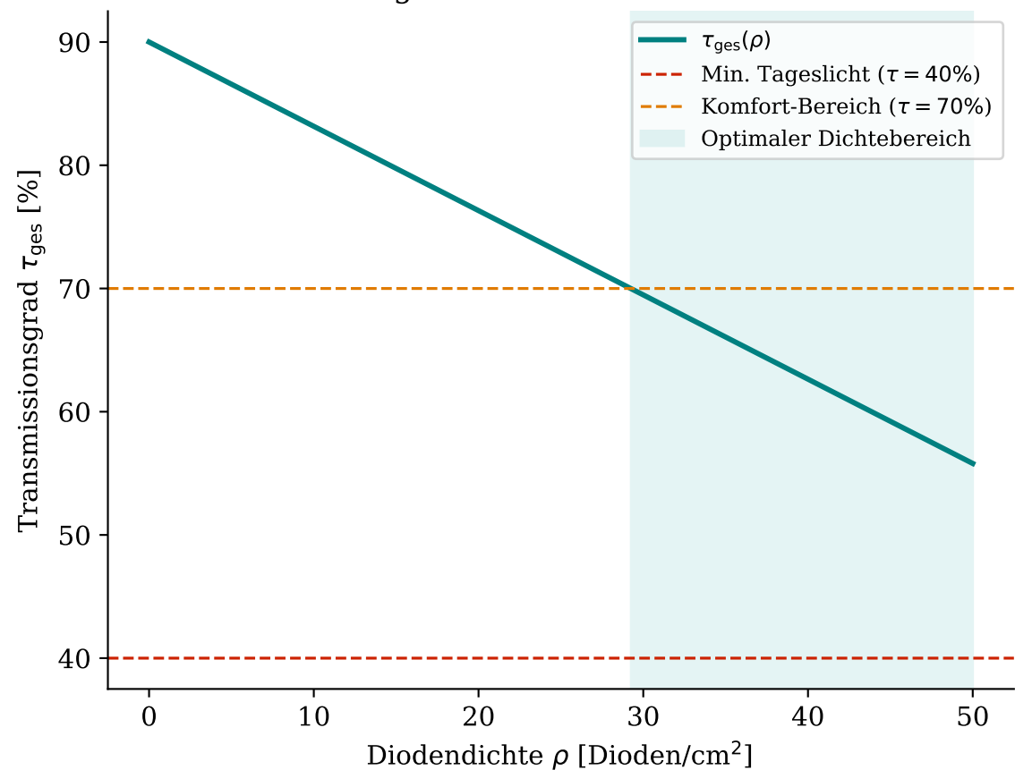
Transmissionsgrad als Funktion der Diodendichte
