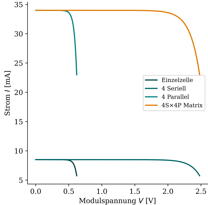
I-V-Kennlinien Verschaltungskonfigurationen
