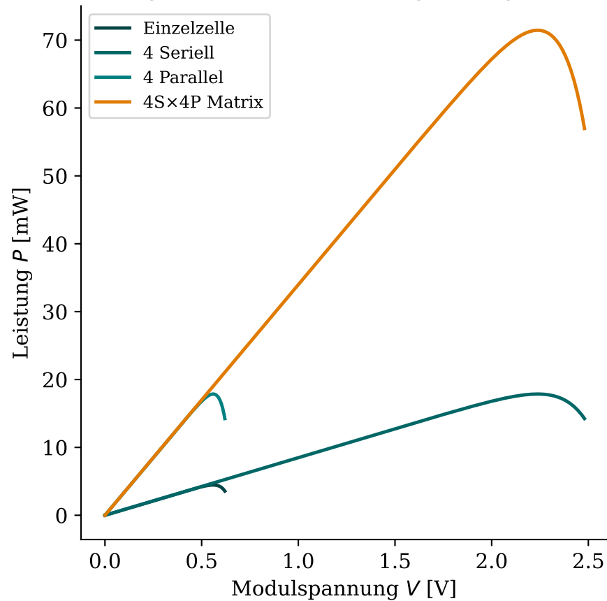
Leistungskurven Verschaltungskonfigurationen
