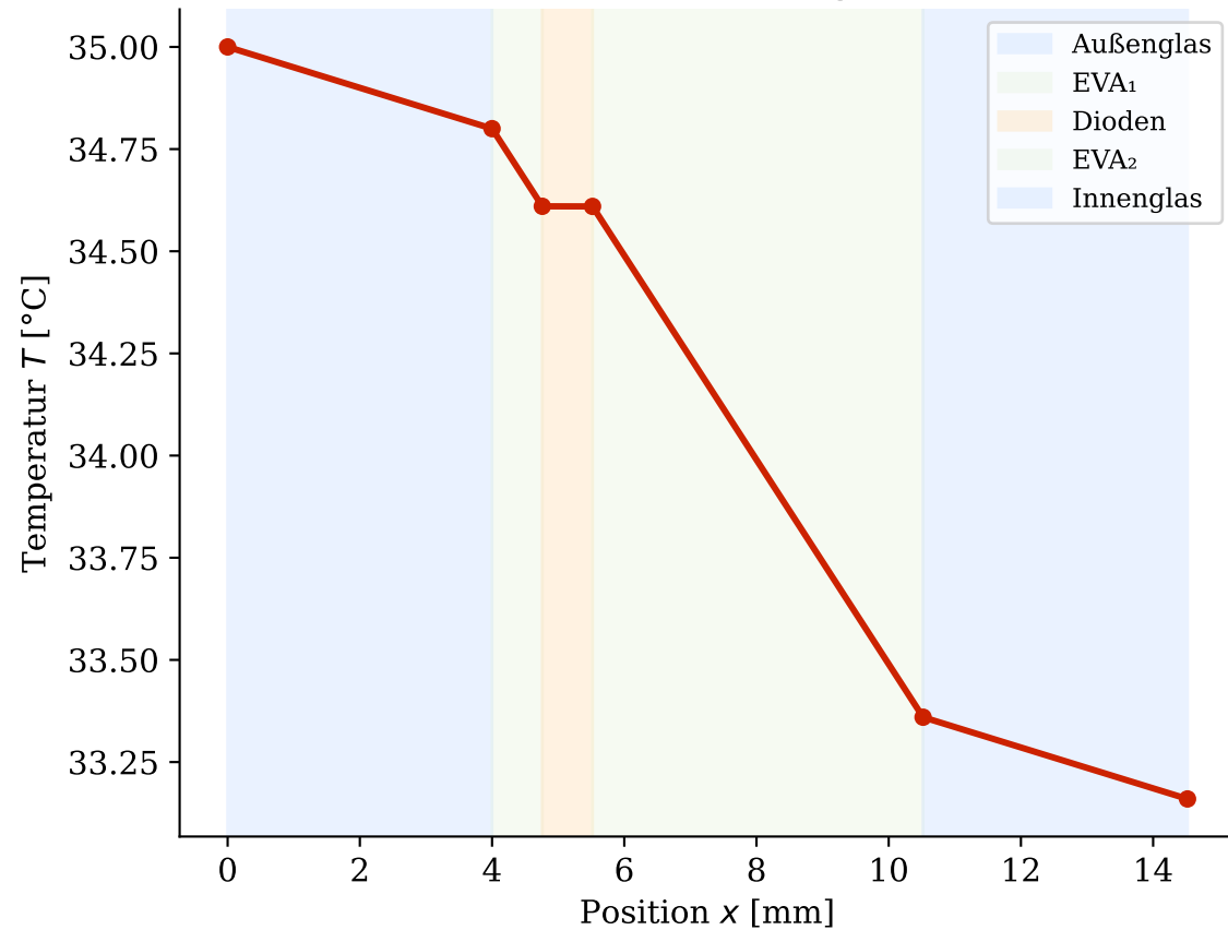
Temperaturprofil im Verbundglas-Querschnitt
