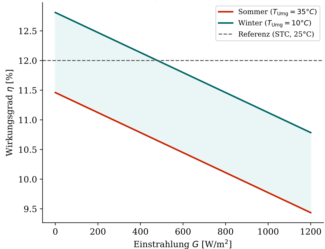
Wirkungsgrad-Temperaturdrift
