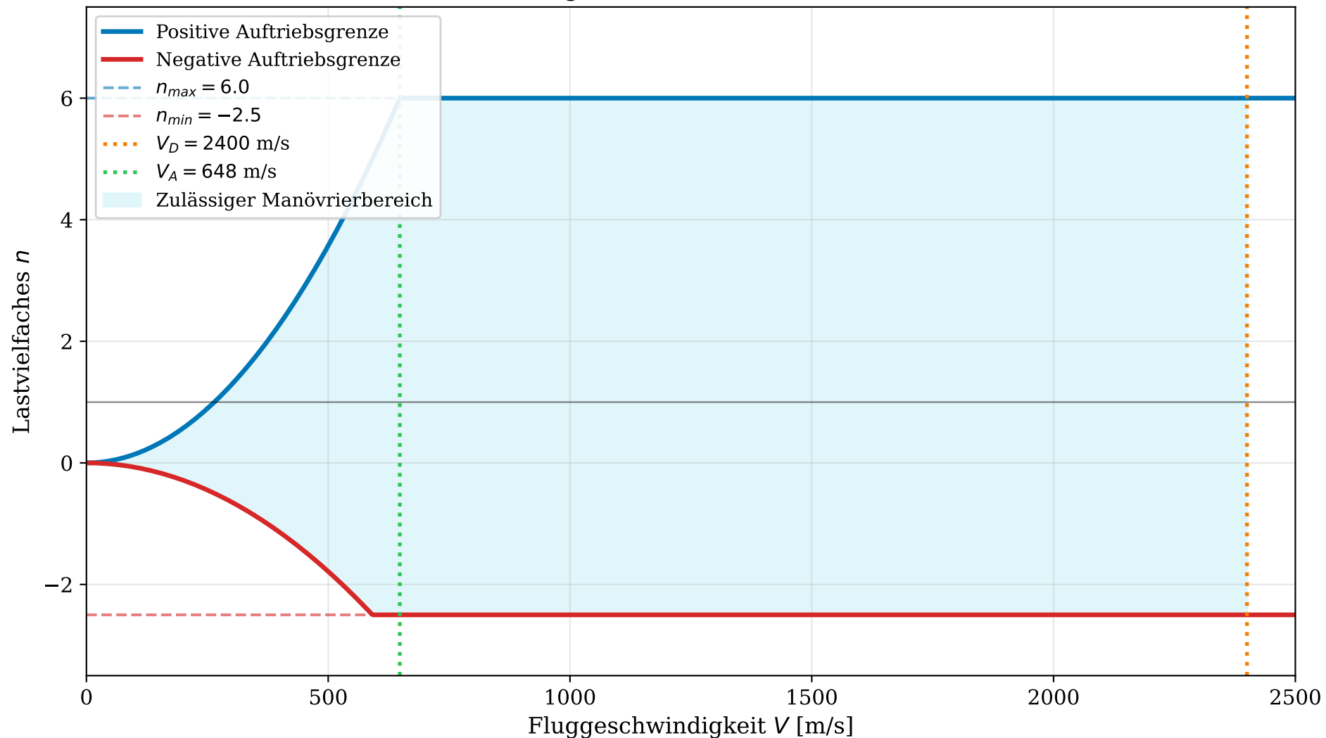
V-n Manövriardiagramm des SR-91 bei H = 20 km (ISA)
