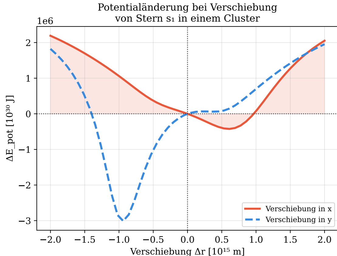
Abbildung 10: Energetische und topologische Auswirkung der Sternverschiebung
