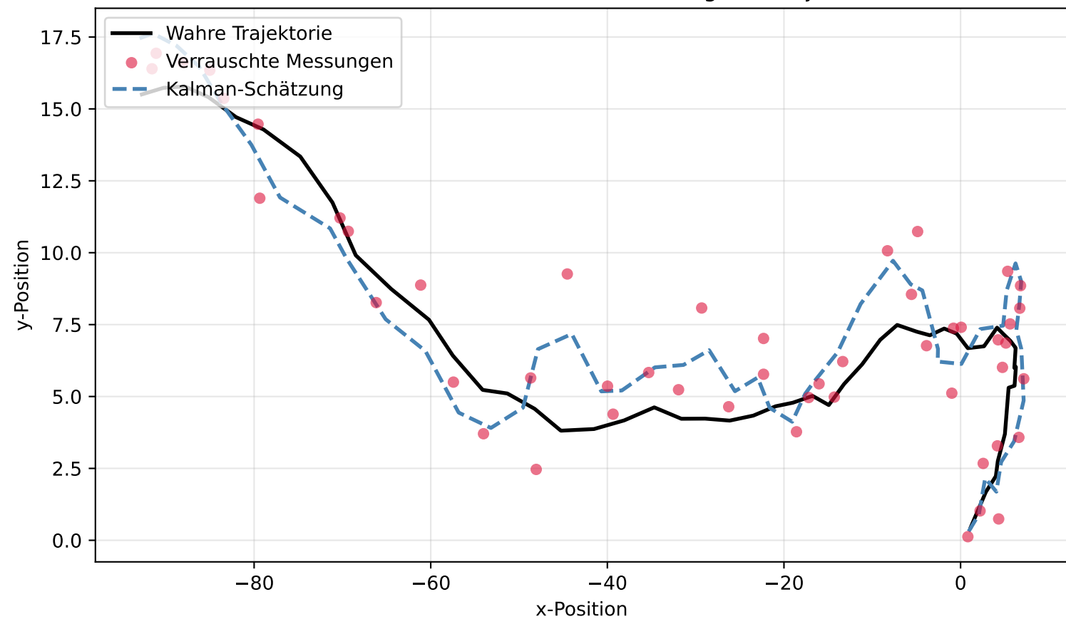
Plot 1: Kalman-Filter Positionsschätzung (2D-Trajektorie)
