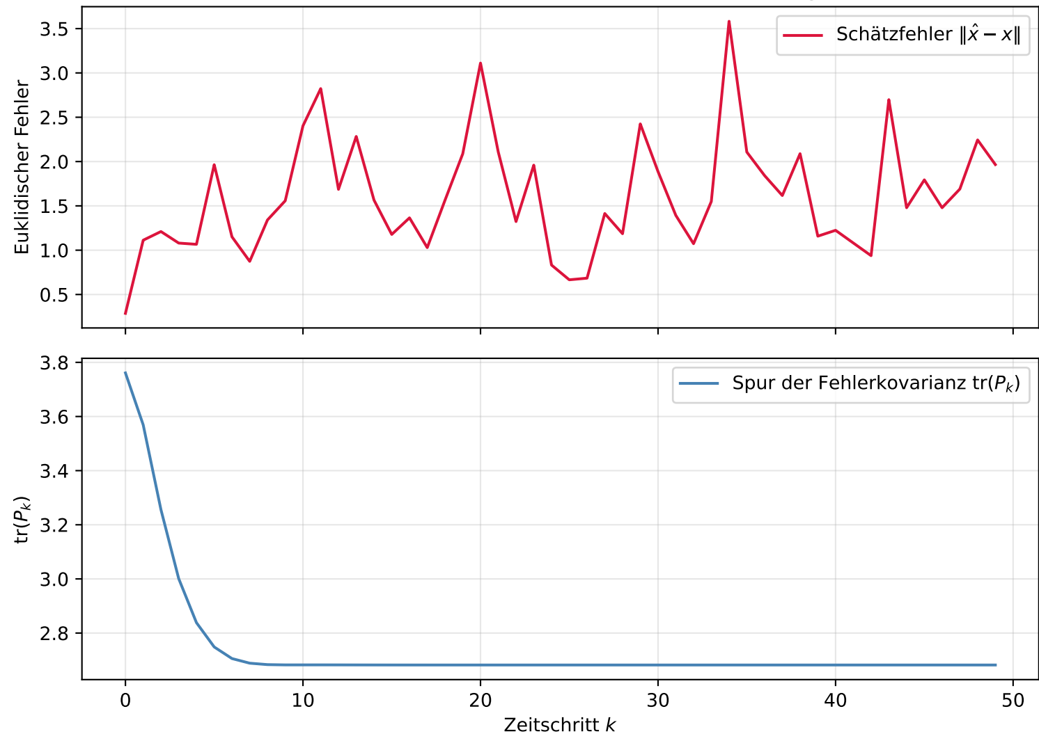
Plot 2: Schätzfehler und Kovarianzentwicklung
