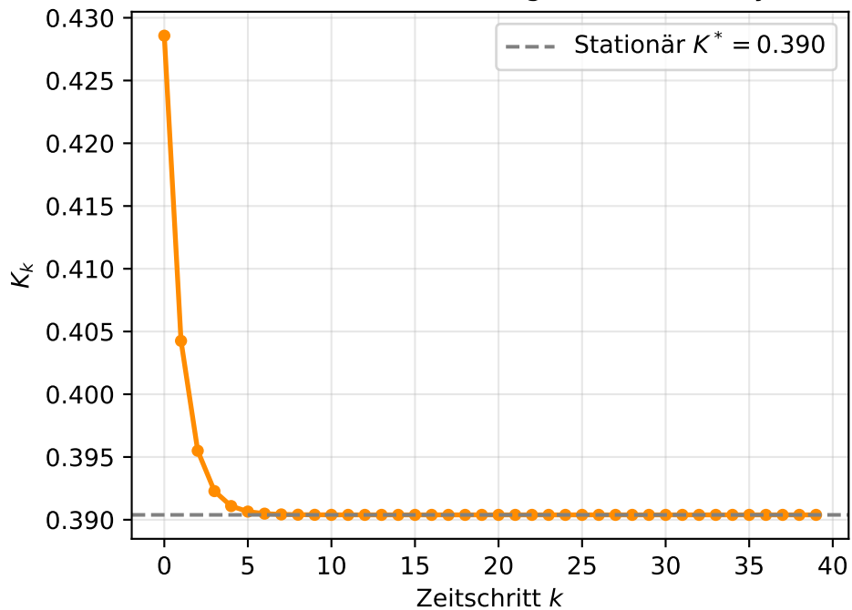
Plot 4a: Kalman-Verstärkung K_k (skalares System)
