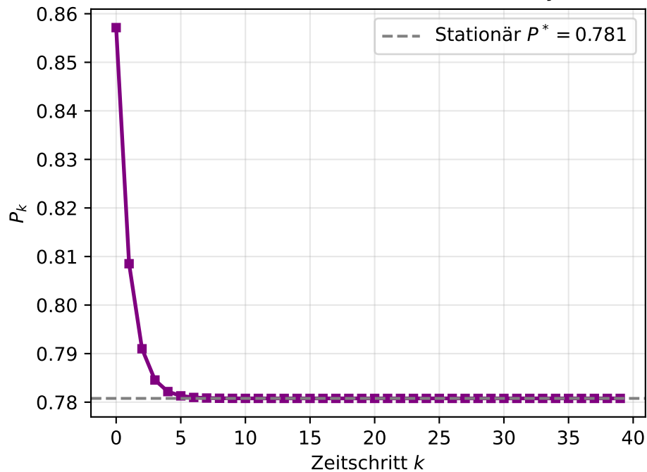
Plot 4b: Fehlerkovarianz P_k (skalares System)
