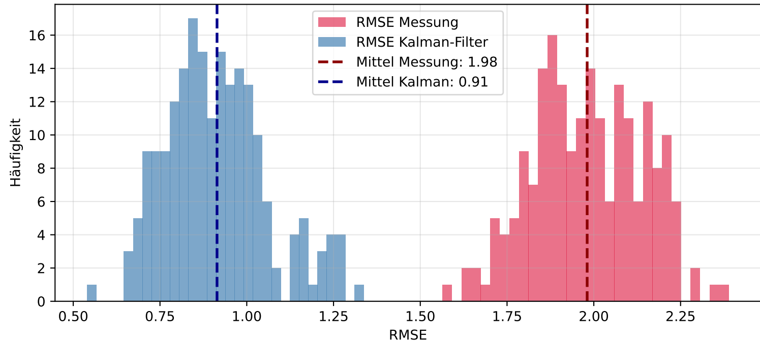
Plot 6: RMSE-Vergleich Kalman-Filter vs. Messung (200 Simulationen)
