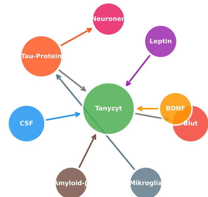
Molekulares Interaktionsnetzwerk: Tanyzyt-Alzheimer-Achse
