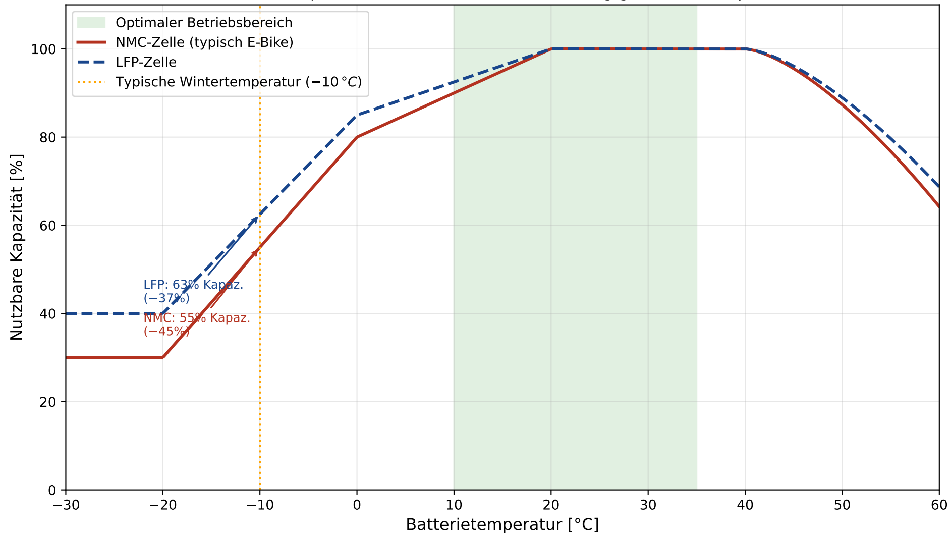
Nutzbare Kapazität von Li-Ion-Akkus in Abhängigkeit der Temperatur
