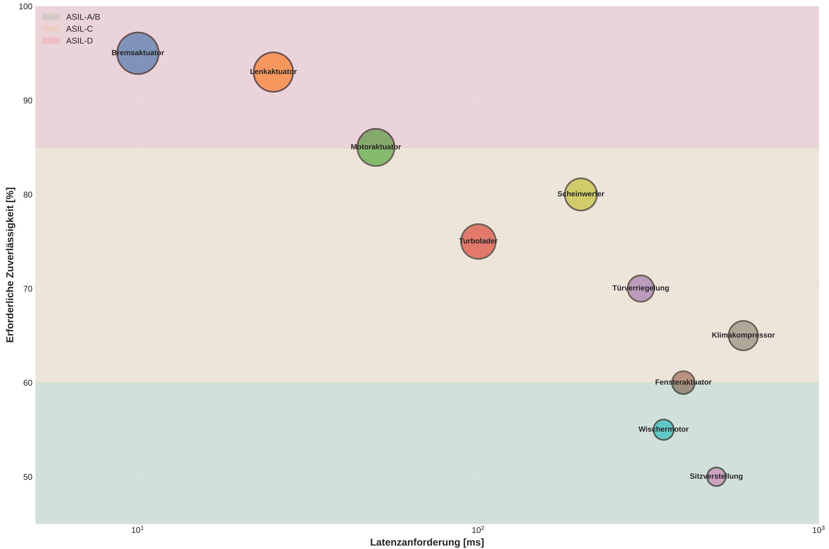
Aktor-Klassifikation: Latenz vs. Zuverlässigkeit vs. ASIL-Level (Bubble-Größe = ASIL-Kritikalität)
