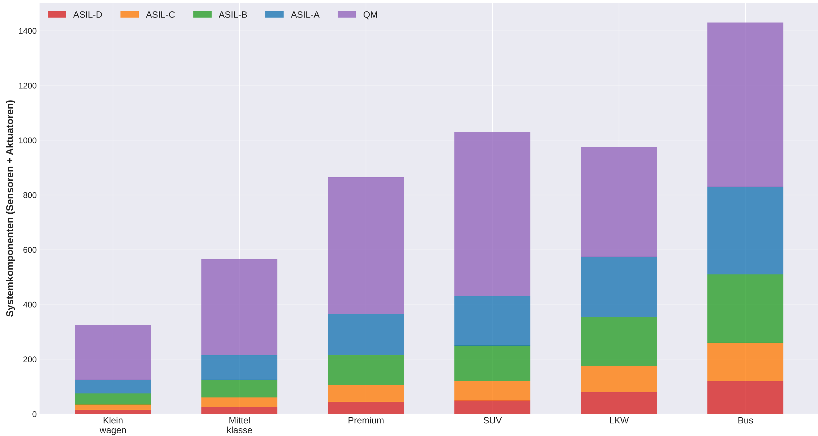
ASIL-Klassifikation nach Fahrzeugtyp und Komplexität
