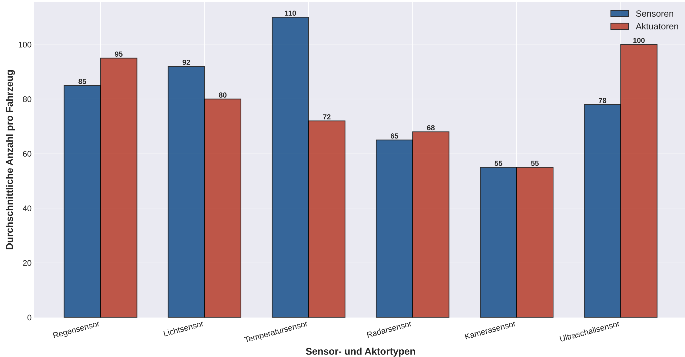
Verteilung von Sensoren und Aktuatoren nach Funktionsgruppe in modernen Kraftfahrzeugen
