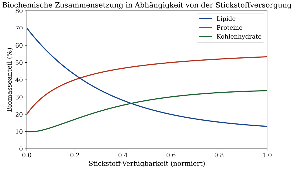
Abbildung 6: Biochemische Zusammensetzung der Algenbiomasse in Abhängigkeit der Stickstoffverfügbarkeit. Bei Stickstoffmangel (links) dominieren Lipide bis zu 70 % der Trockenmasse, was für Biokraftstoffanwendungen genutzt wird. Bei ausreichender Stickstoffversorgung (rechts) steigt der Proteingehalt auf über 50 %, was für Futter- und Lebensmittelanwendungen relevant ist.
