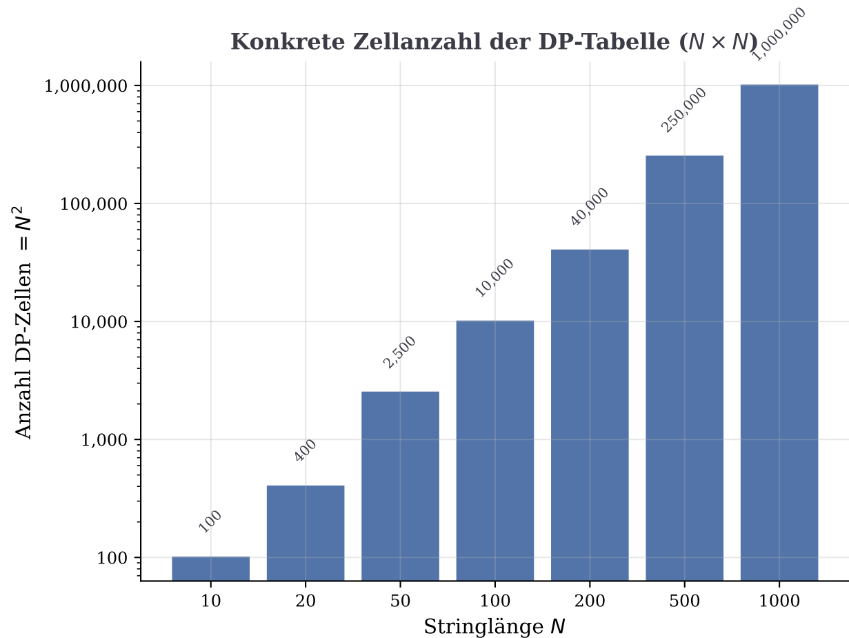
Abbildung 2: Quadratische Laufzeitkomplexität der Dynamischen Programmierung – \mathcal{O}(N^2)
